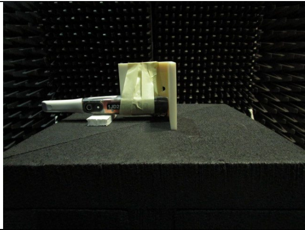
Horizontal EUT
