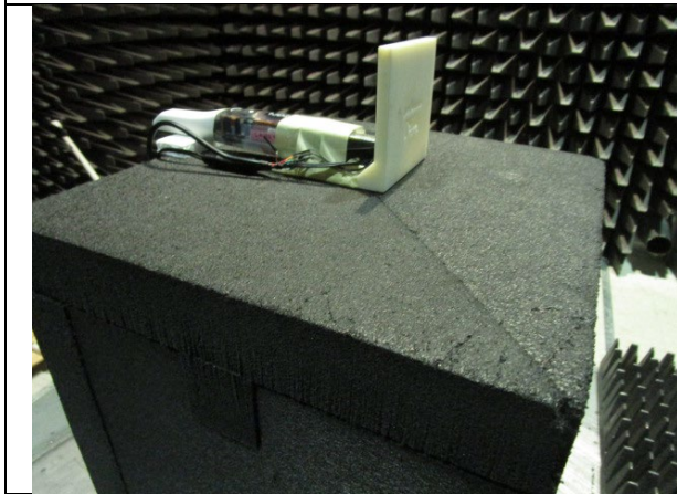
Flat EUT
