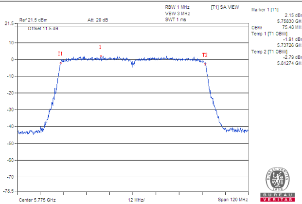
802.11ac (VHT80+VHT80) / Chain 2 / CH 42+155
