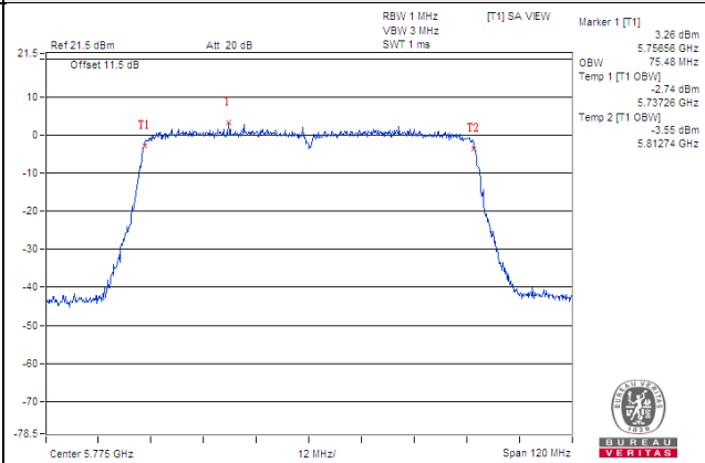
802.11ac (VHT80+VHT80) / Chain 3 / CH 42+155
