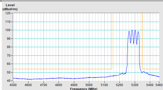
Vertical (Average)
