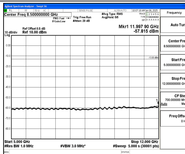
Band25-10MHz-QPSK-26365-1-0-Low-5000-12000--57.82-PASS
