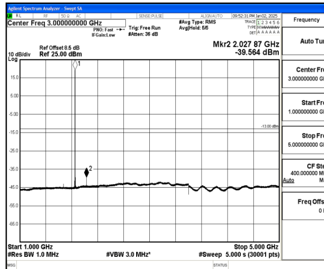
Band25-20MHz-QPSK-26140-1-0-Low-1000-5000--39.56-PASS
