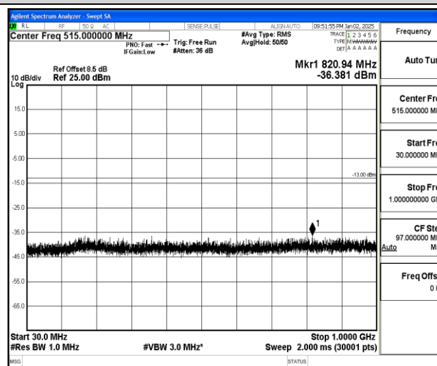
Band25-20MHz-QPSK-26140-1-0-Low-30-1000--36.38-PASS
