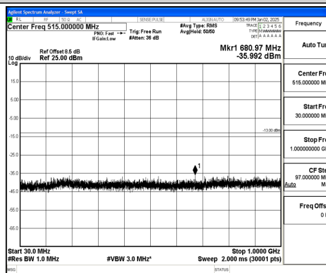
Band25-20MHz-16QAM-26140-1-0-Low-30-1000--35.99-PASS
