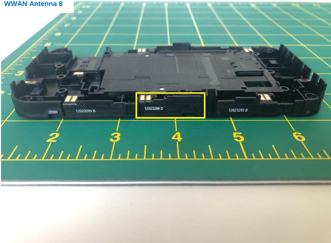
WWAN Antenna 8
