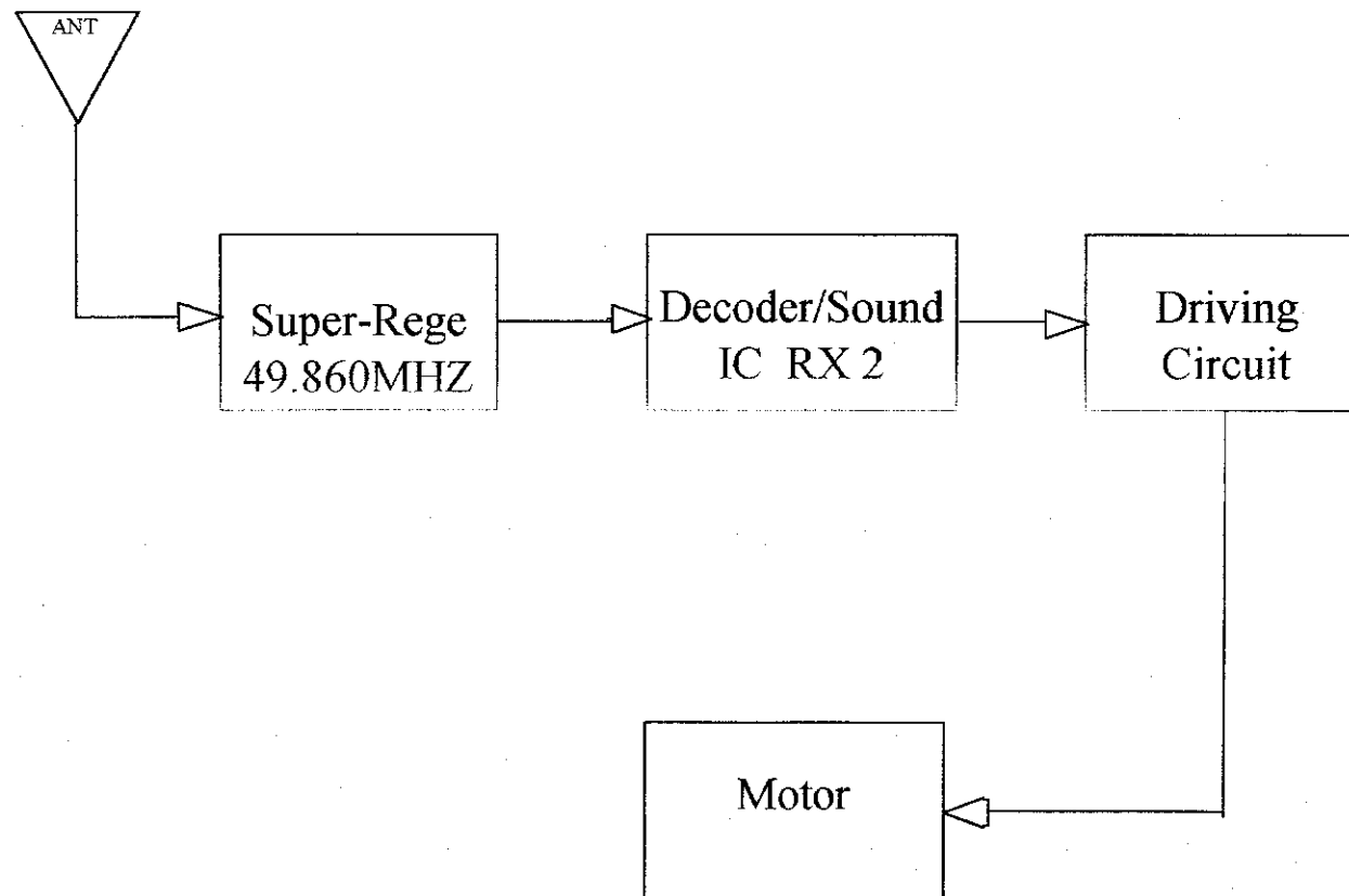
橢圓桶形電單車/遙控車49MHz RX 方框圖
