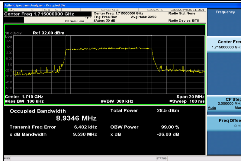
Band4-10MHz-QPSK-20000-50RB#0-8.9346
