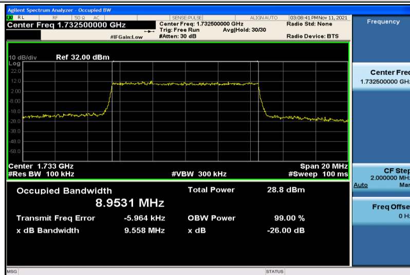
Band4-10MHz-QPSK-20175-50RB#0-8.9531
