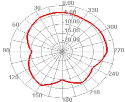
940.000MHz E2
