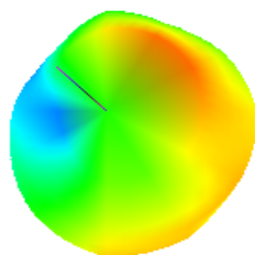
940.000MHz
