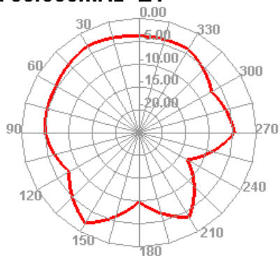
700.000MHz E1
