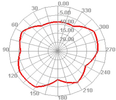
840.000MHz E2
