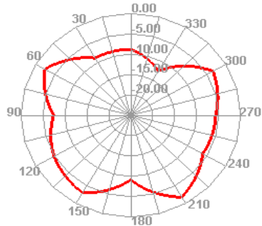
840.000MHz E1
