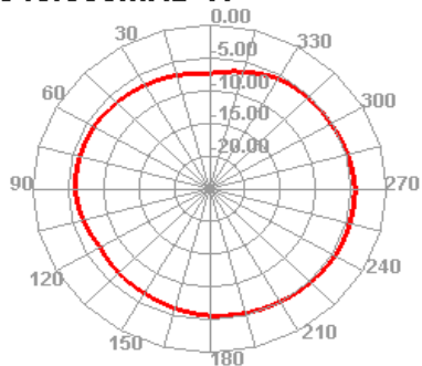
840.000MHz H
