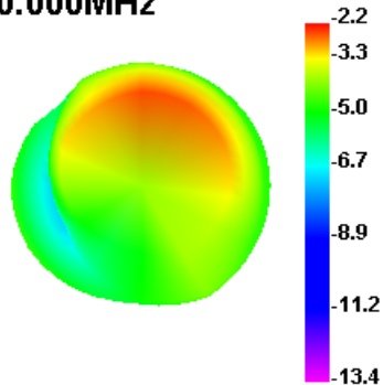
700.000MHz E1
