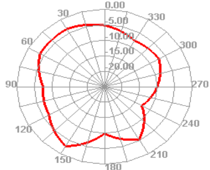
940.000MHz E1
