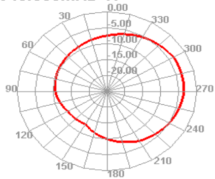
940.000MHz H
