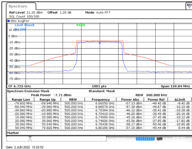
802.11ax (40MHz) / 6725MHz / Chain A / NSS-4
