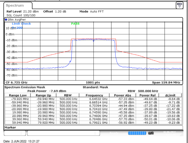
802.11ax (40MHz) / 6725MHz / Chain D / NSS-4
