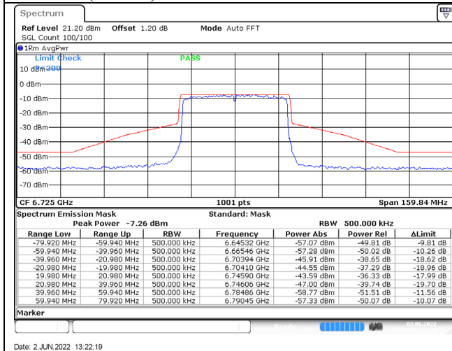
802.11ax (40MHz) / 6725MHz / Chain C / NSS-4
