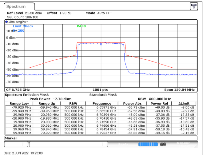
802.11ax (40MHz) / 6725MHz / Chain B / NSS-4
