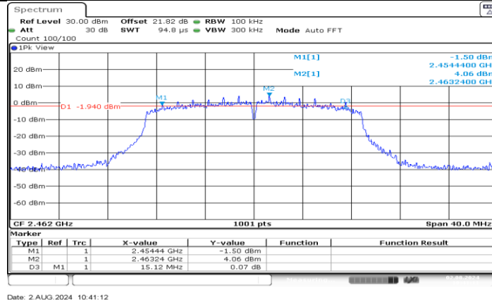
11N20SISO_Ant2_2462
