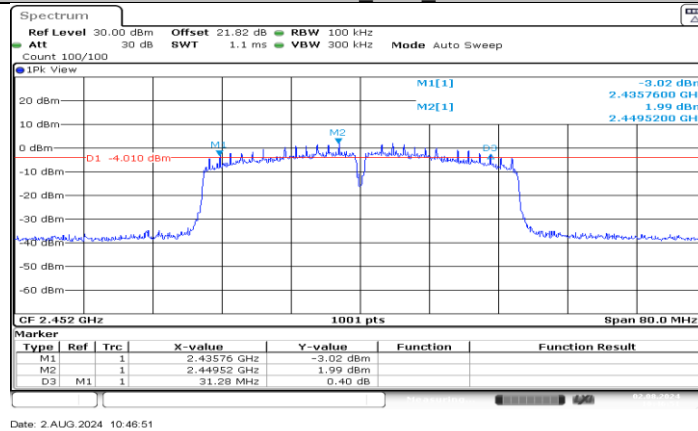
11N40SISO_Ant2_2452
