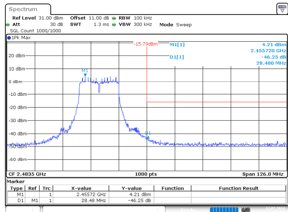
n20_2462MHz_Chain 0
