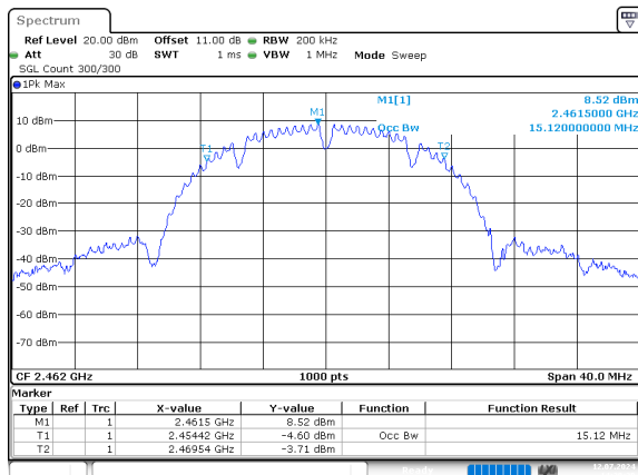
b_2462MHz_Chain 0
