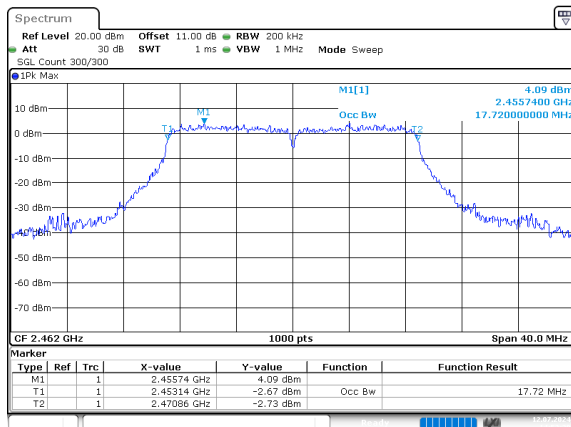
n20_2462MHz_Chain 0
