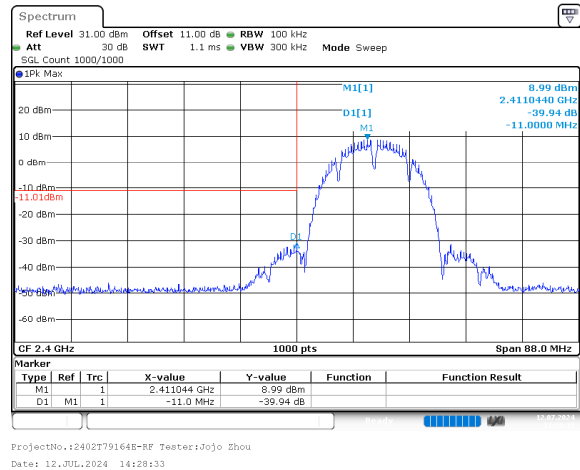
b_2412MHz_Chain 0
