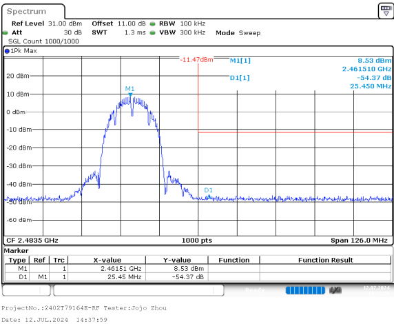
b_2462MHz_Chain 0
