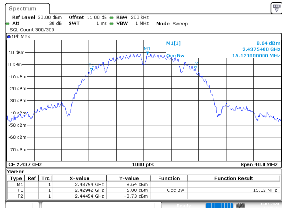
b_2437MHz_Chain 0
