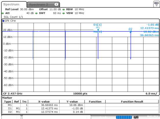
b_2437MHz_Chain 0
