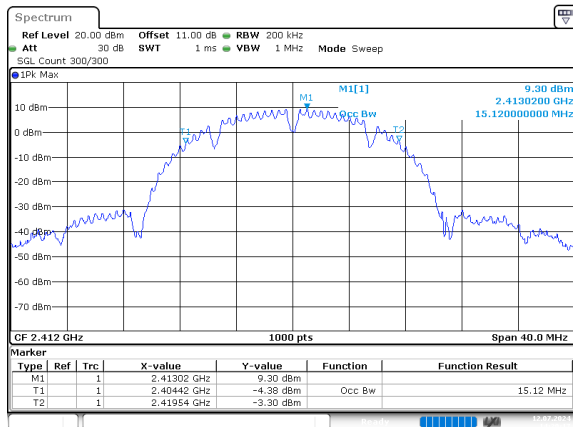
b_2412MHz_Chain 0
