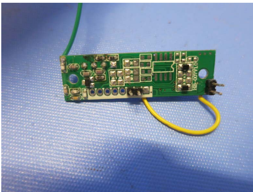
Tx module PCB comp side
