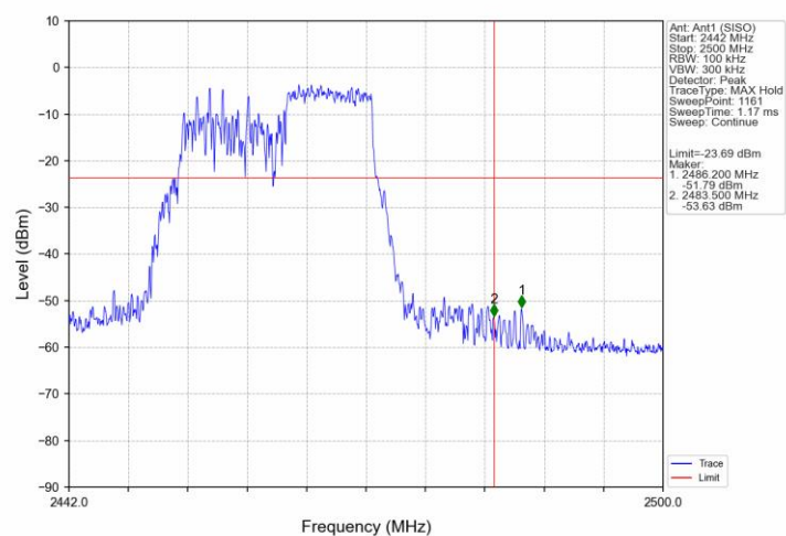
802.11ax(HEW20)_HCH_2462MHz_RU242_61_Ant1 (SISO)_NTNV
