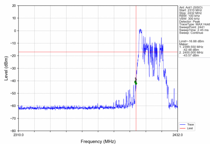
02.11ax(HEW20) LCH_2412MHz_RU52_37_Ant1 (SISO)_NTNV
