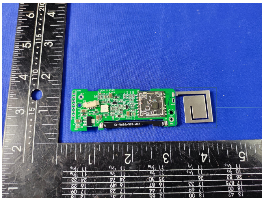
LORA ANTENNA
