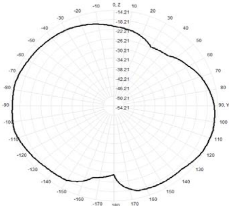
905.0MHz Total(E2-YZ), Max= -14.66dBi
