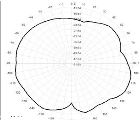
922.0MHz Total(E1-XZ), Max= -11.54dBi
