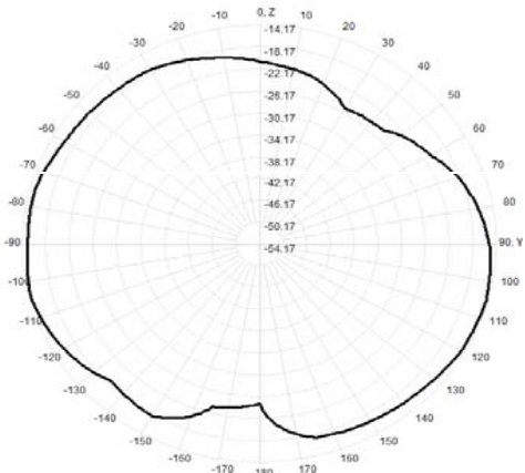
906.0MHz Total(E2-YZ), Max= -14.49dBi
