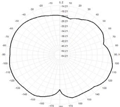
905.0MHz Total(E1-XZ), Max= -14.21dBi
