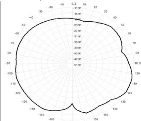
920.0MHz Total(E1-XZ), Max= -11.91dBi
