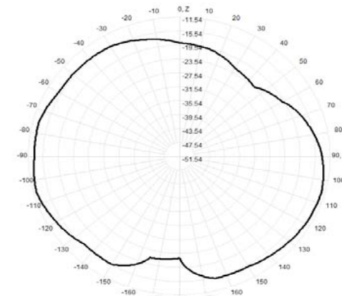
922.0MHz Total(E2-YZ), Max= -12.40dBi
