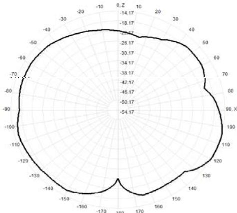
906.0MHz Total(E1-XZ), Max= -14.17dBi
