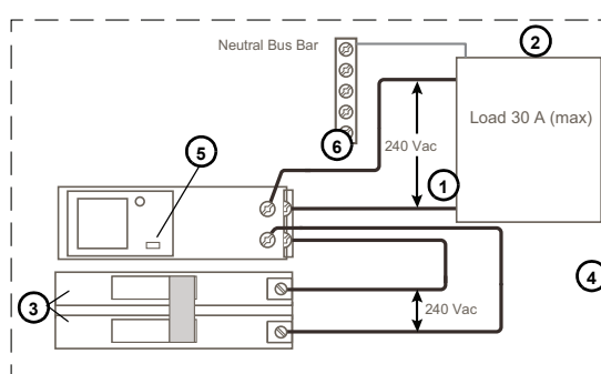
Figure / Figura / Figure 2 : Installation Diagram / Diagrama de instalación / Schéma d'installation
