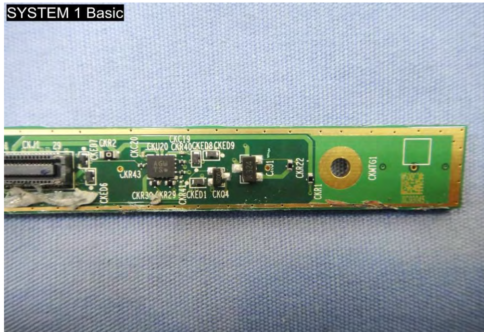
EUT Photo (74)
