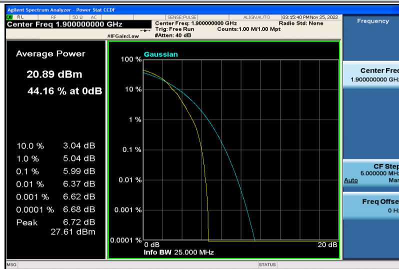
Band2-20MHz-64QAM-19100-1RB#0
