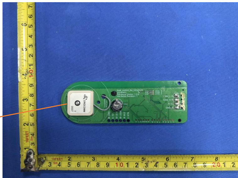
GPS ANT
