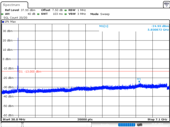
5MHz_Middle_QPSK_25@0 -24.93dBm
