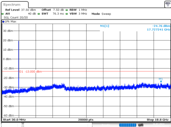
20MHz_Middle_QPSK_1@0 -24.76dBm
