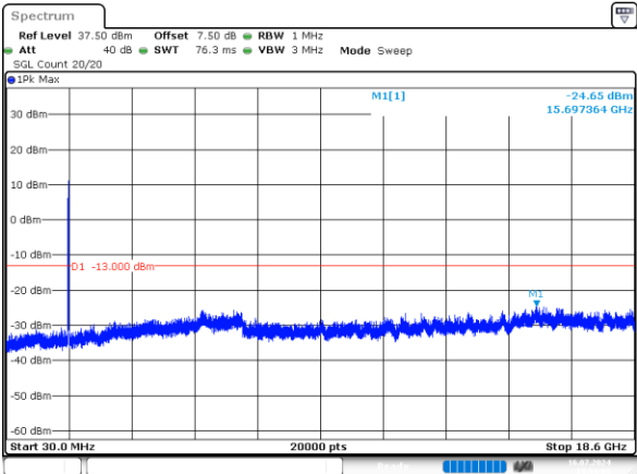
20MHz_Low_QPSK_100@0 -24.65dBm
