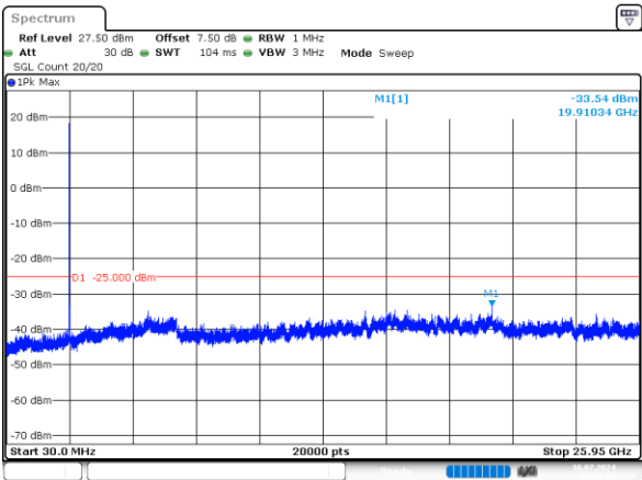
5MHz_Middle_QPSK_25@0 -33.54dBm
