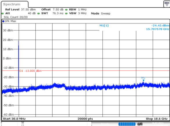
20MHz_Low_QPSK_1@0 -24.45dBm
