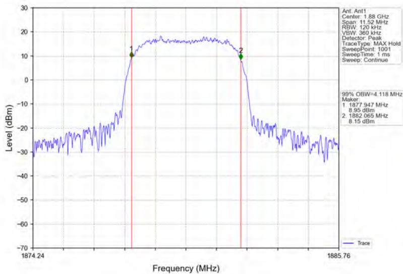
Band2_HSUPA_MCH_1880MHz_Subtest 1_NTNV
