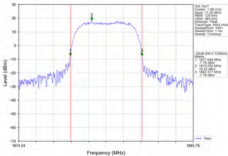
Band2_HSUPA_MCH_1880MHz_Subtest 1_NTNV
