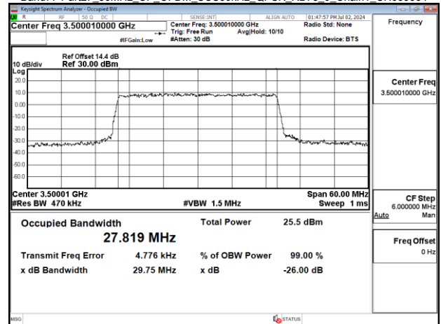
Band77-Part27_30MHz_CP_OFDM_SCS30kHz_QPSK_RB78_0_Chain1_CH633334
