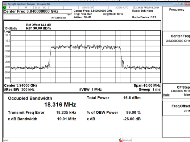
Band77-Part27_20MHz CP OFDM SCS30kHz 256QAM RB51_0 Chain1_CH656000
