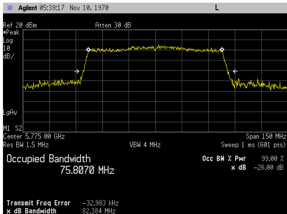
p20c0005_99%_80MHZ_UNII-3_AC_P1
