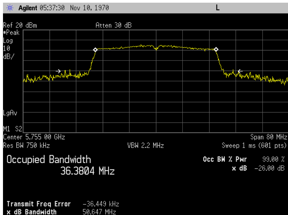
p20c0005_99%_40MHZ_Low Channel_UNII-3_AC_P1
