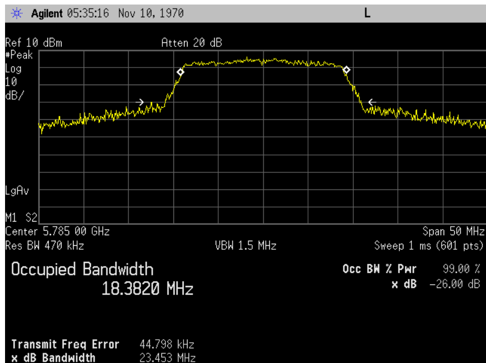
p20c0005_99%_20MHZ_Mid Channel_UNII-3_AC_P1
