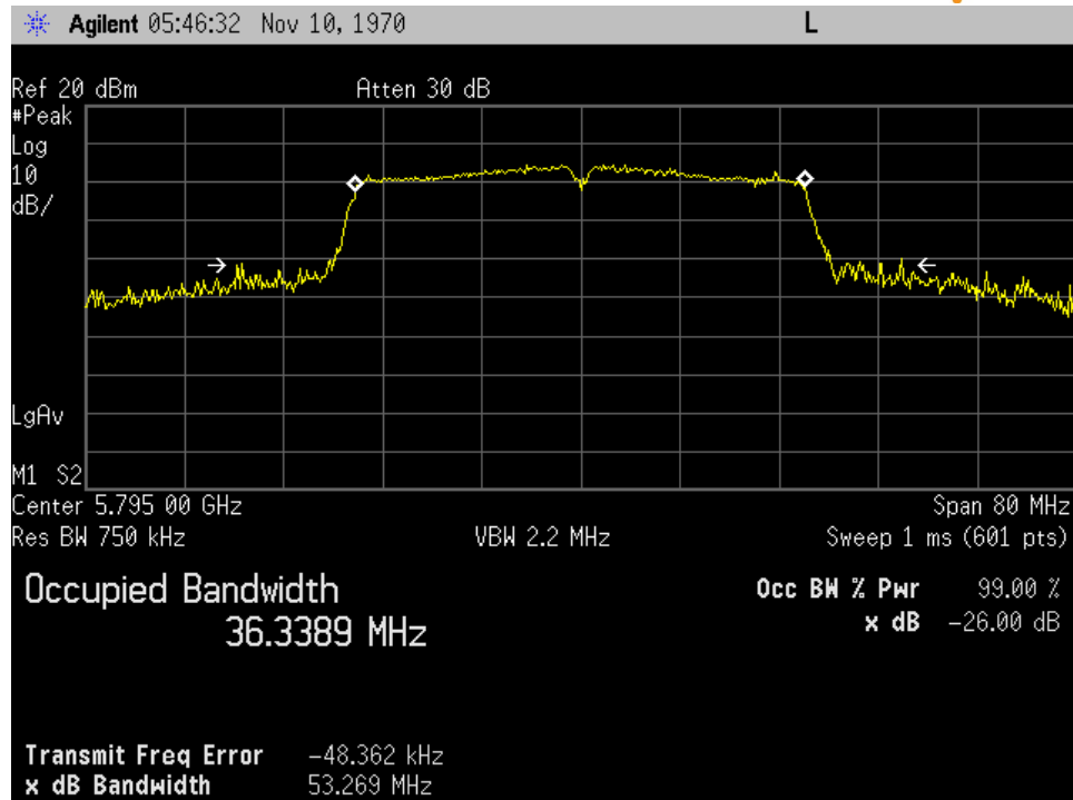
p20c0005_99%_40MHZ_High Channel_UNII-3_AC_P1
