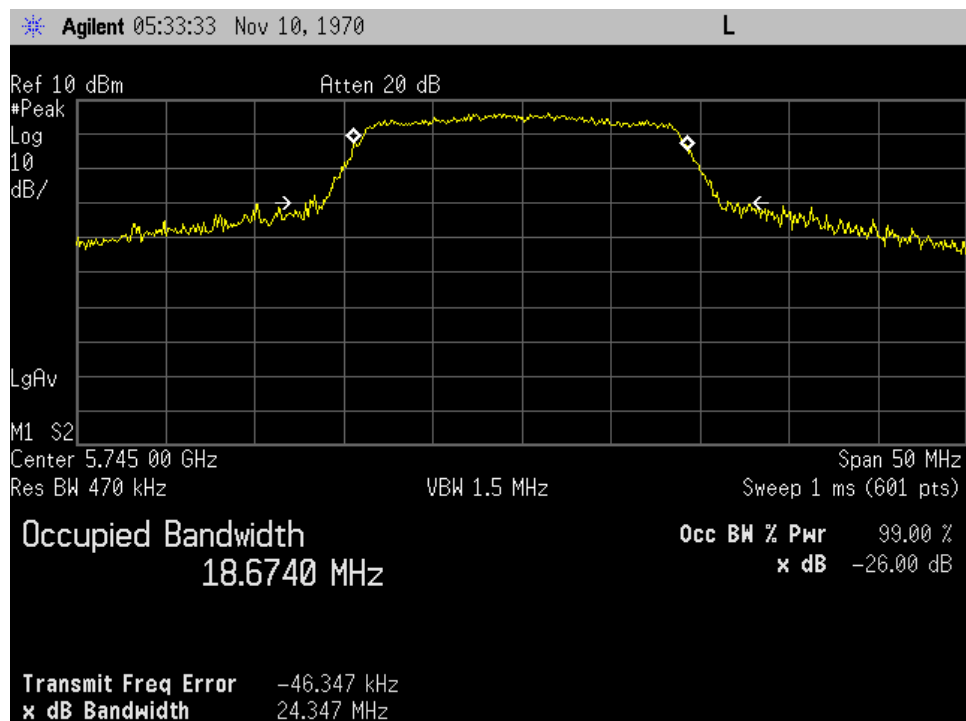
p20c0005_99%_20MHZ_Low Channel_UNII-3_AC_P1
