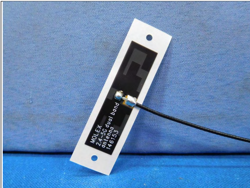
Antenna 10 (Brand: MOLEX ; Model: 1461530100)
