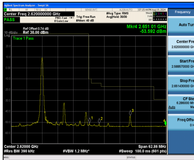
Band38-20MHz-QPSK-38150-1RB#99
