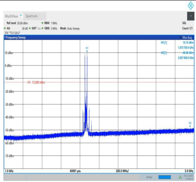
2-2-20MHz-5MHz-QPSK-QPSK-18700-18817-1RB#0-1RB#24 -1000~3000MHz-PASS
