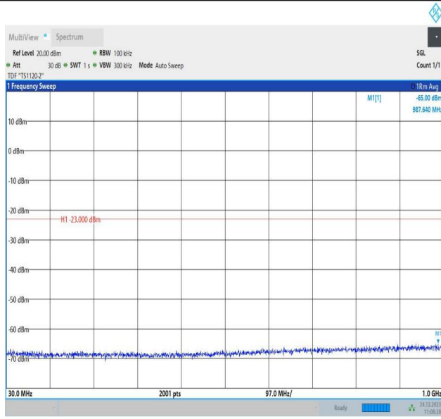
2-2-20MHz-5MHz-QPSK-QPSK-18700-18817-1RB#0-1RB#24 -30~1000MHz-PASS
