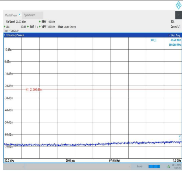
2-2-20MHz-5MHz-QPSK-QPSK-18700-18817-100RB#0-25RB #0-30~1000MHz-PASS
