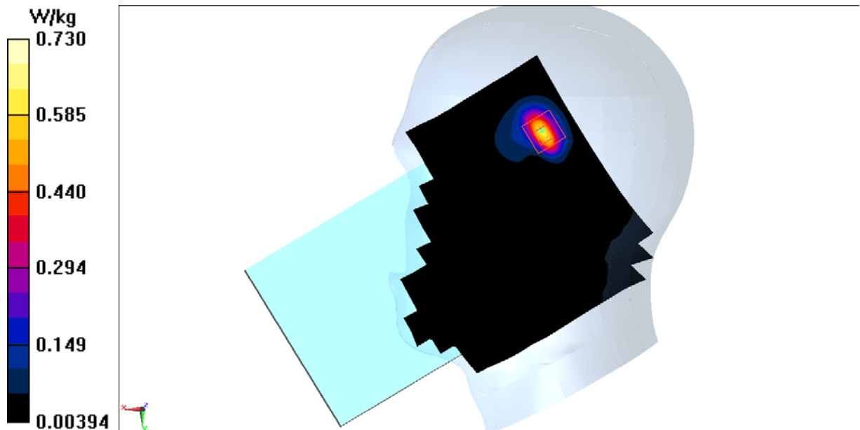
Fig. 17 LTE Band 7
