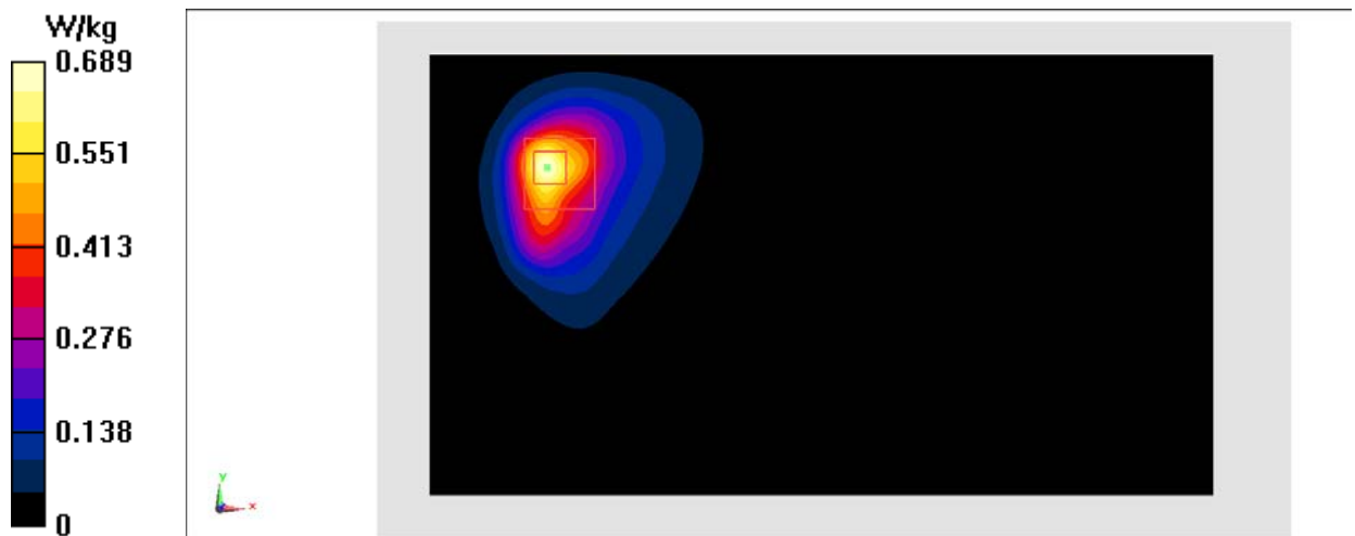
Fig.6 WCDMA 850
