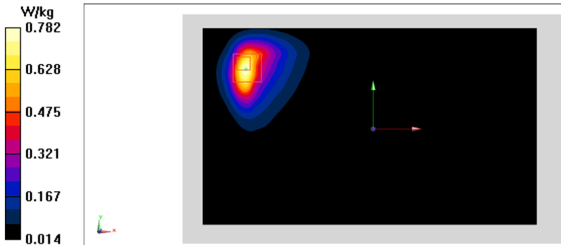
Fig.16 LTE Band5
