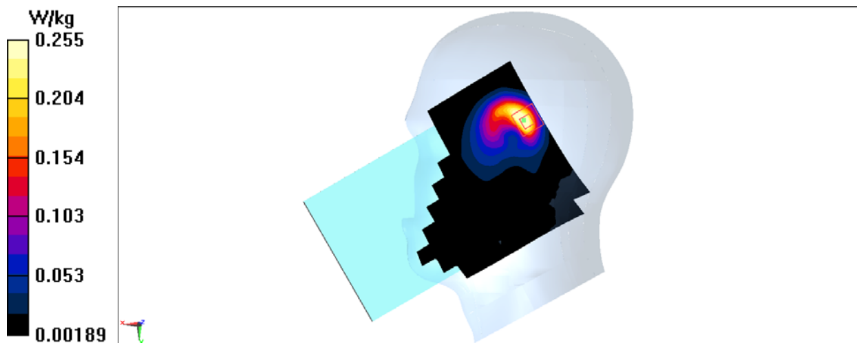
Fig.9 WCDMA1900
