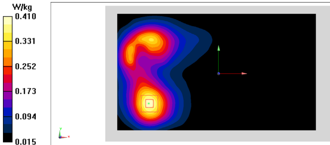
Fig.10 WCDMA1900
