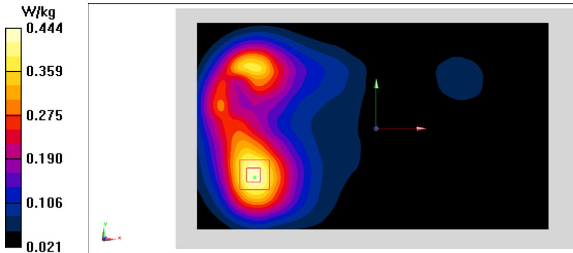
Fig.8 WCDMA1700
