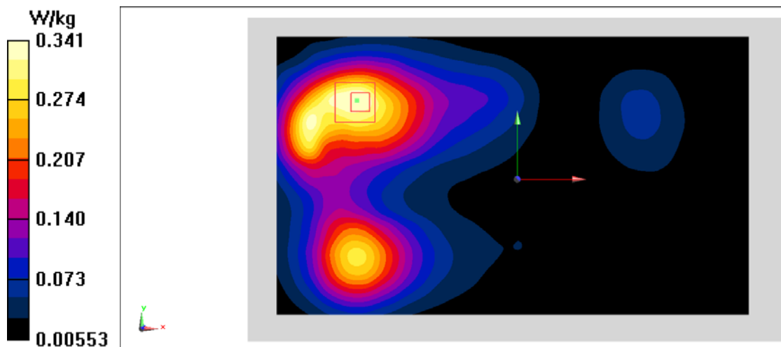
Fig.12 LTE Band2
