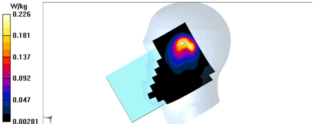
Fig.7 WCDMA1700
