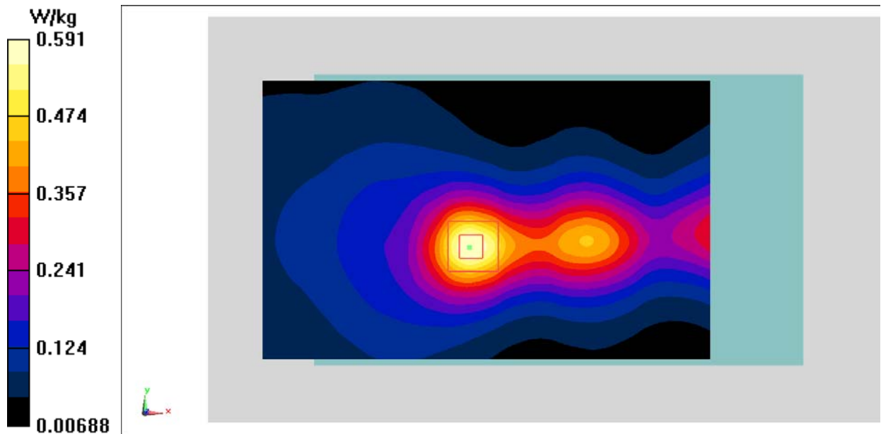
Fig. 18 LTE Band 7
