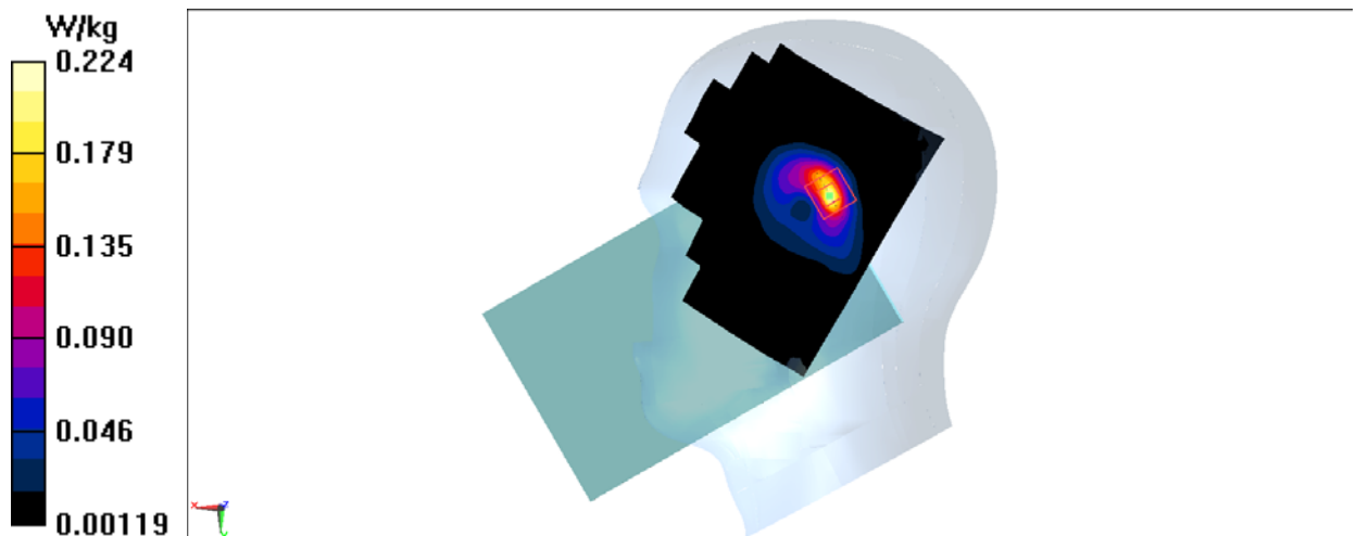
Fig.11 LTE Band2
