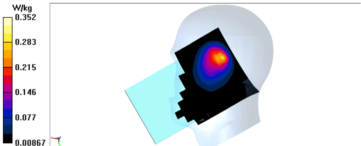
Fig.15 LTE Band5
