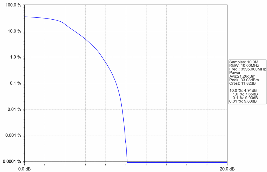
Band42c 10MHz QPSK HCH 3595MHz RB 50 0 NTNV
