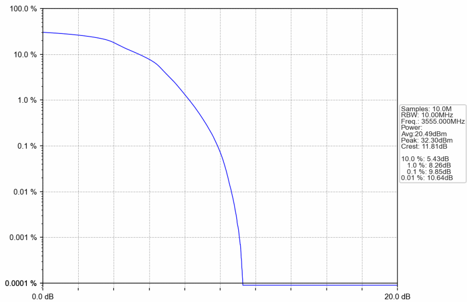
Band42c 10MHz 16QAM LCH 3555MHz RB 50 0 NTNV
