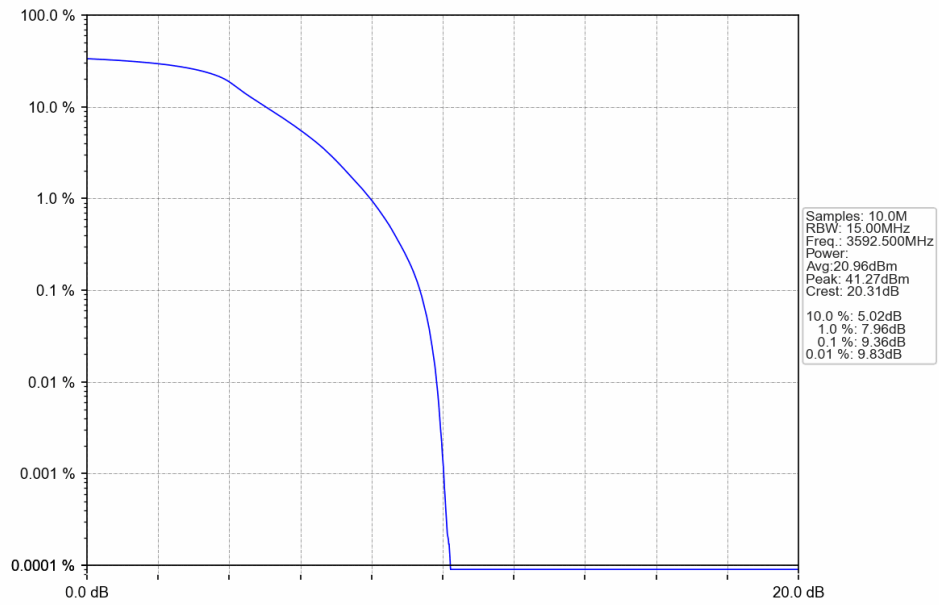
Band42c 15MHz QPSK HCH 3592.5MHz RB 75 0 NTV
