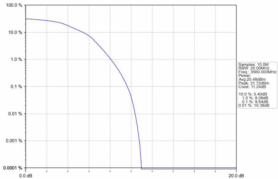
Band42c 20MHz 16QAM LCH 3560MHz RB 100 0 NTNV
