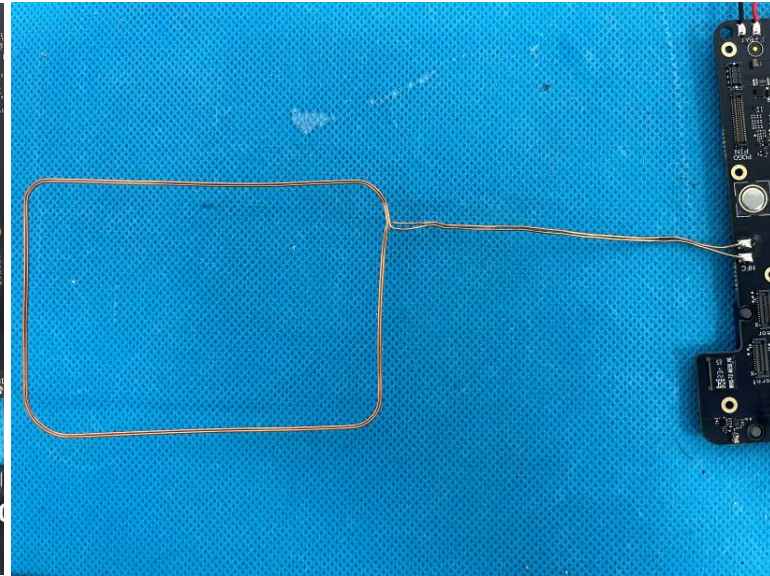
NFC Antenna
