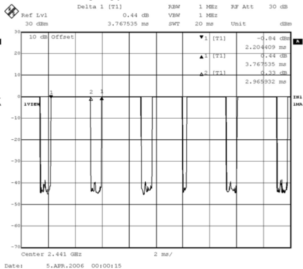
CH 39 2441MHz
