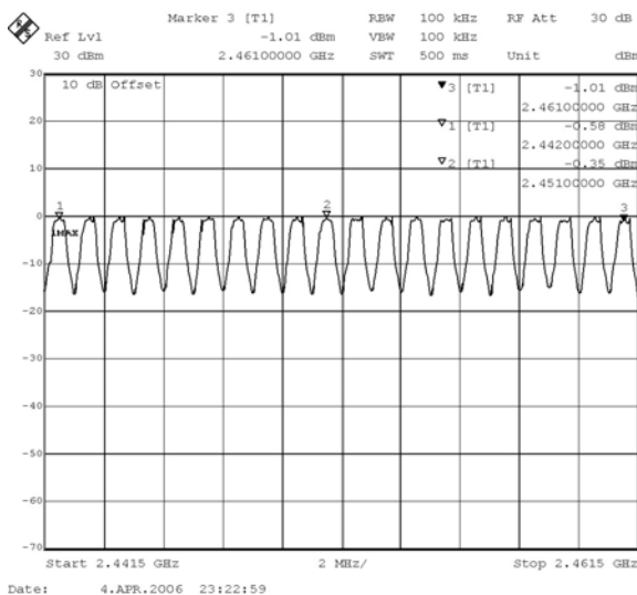
2442-2461MHz
