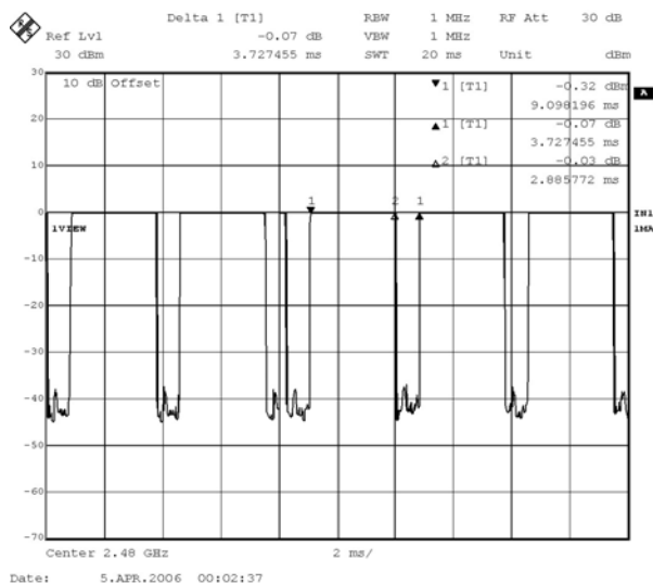
CH 78 2480MHz
