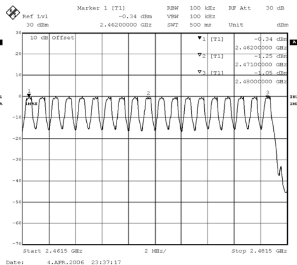
2462-2481MHz
