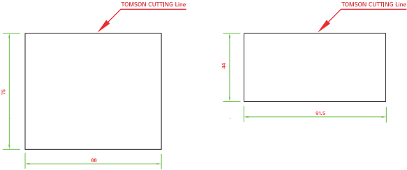
DIE CUT / DIMENTION
