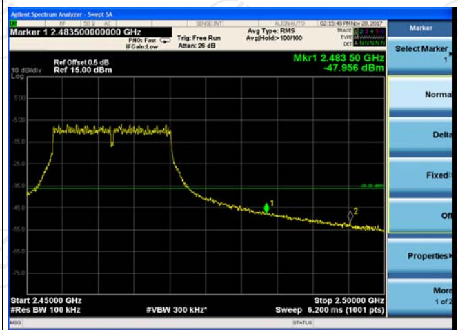
Band Edge
