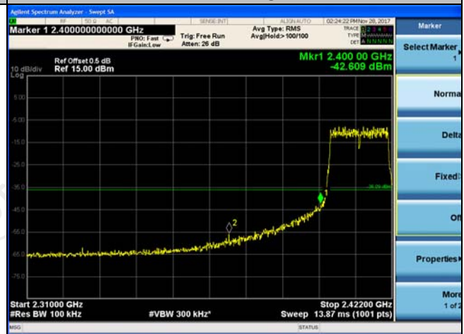
Band Edge
