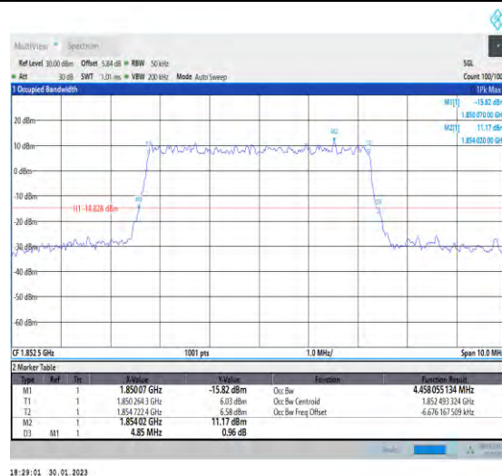
1-N2-PC3-15-5-L-4-DFT-64QAM-Outet_Full-25@0-A nt1-4.458-4.850-≤5-PASS
