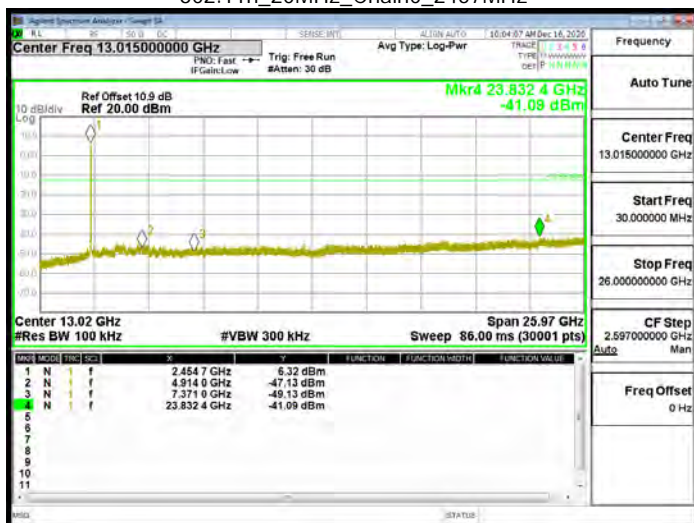
802.11n_20MHz_Chain0_2457MHz
