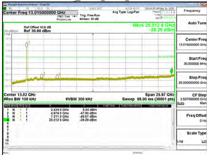
802.11g_20MHz_Chain0_2437MHz
