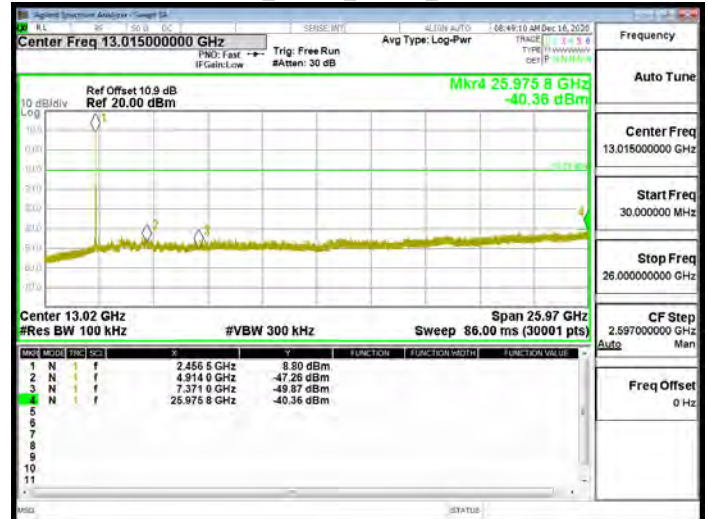
802.11b_20MHz_Chain0_2462MHz
