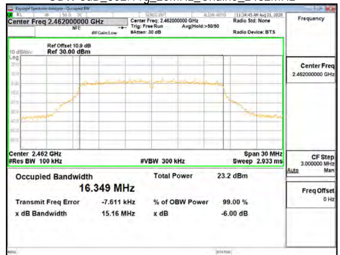
OBW 6dB_802.11g_20MHz_Chain0_2462MHz
