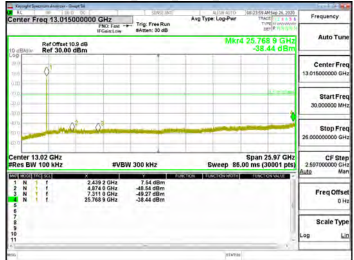
802.11b_20MHz_Chain0_2457MHz
