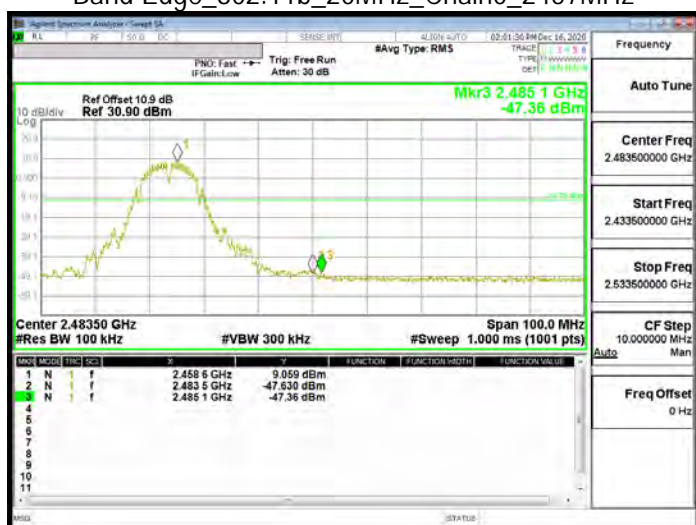
Band Edge_802.11b_20MHz_Chain0_2457MHz
