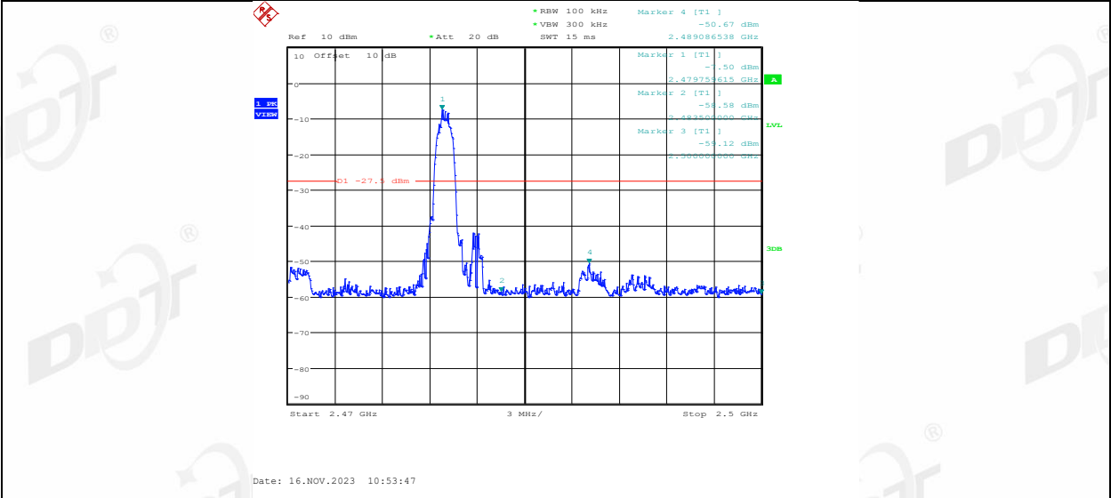
2DH5_Ant2_Low_Hop_2402
