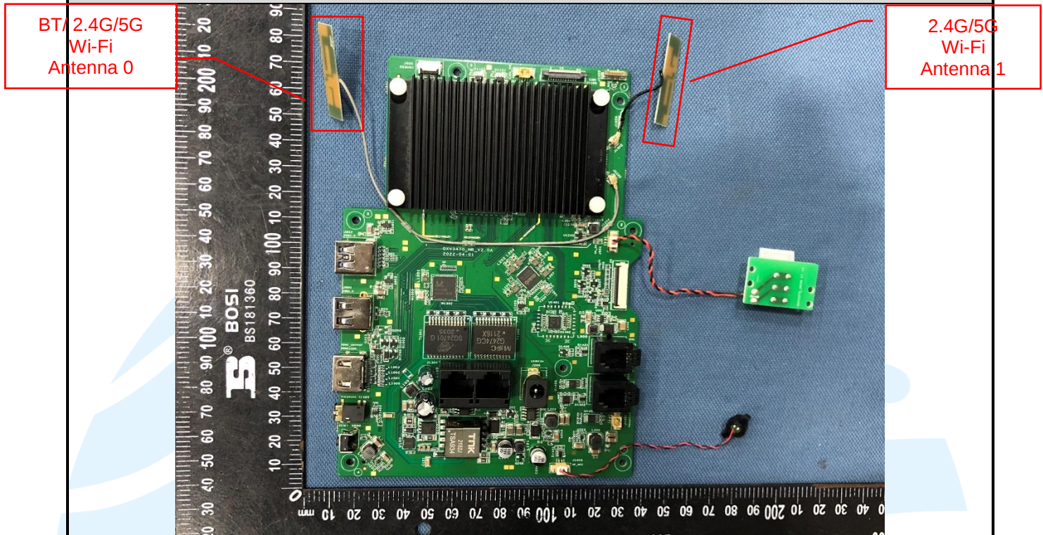
EUT Photo
