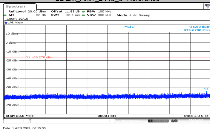
LE 2M_Ant1_2440_30~1000
