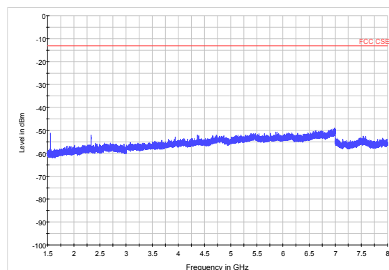
LTE Band 13 10MHz CH-Middle 1.5GHz~8GHz
