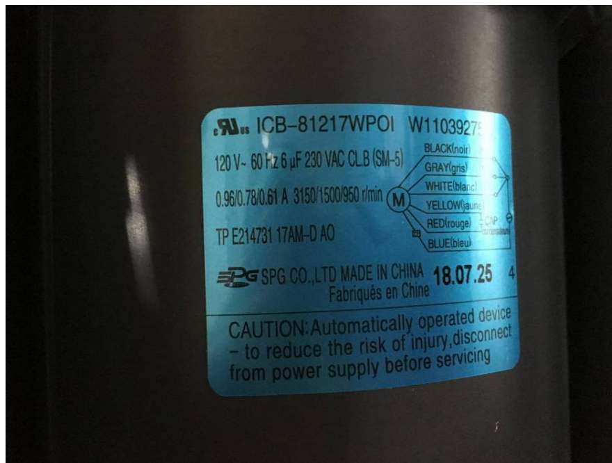
EUT – Fan 2 Label View
