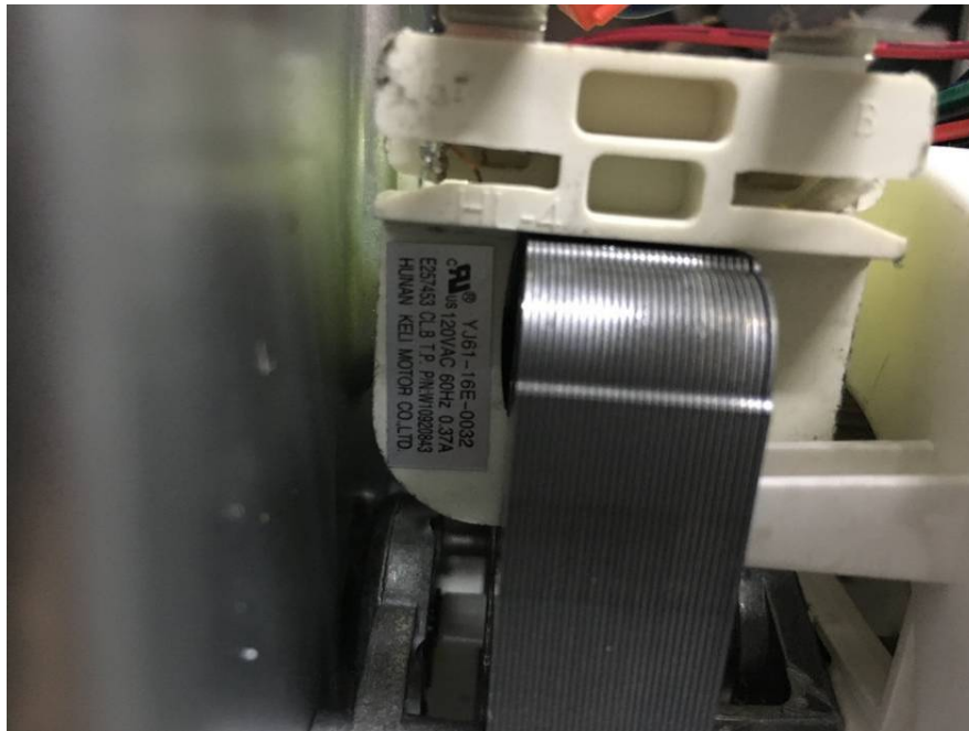
EUT – Fan 1 Label View
