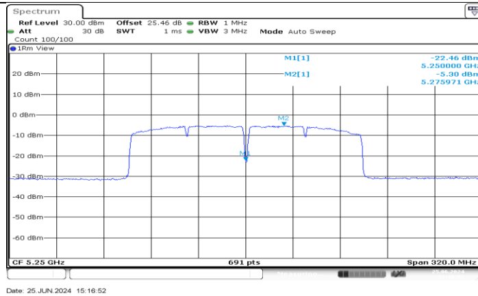
11AC160MIMO_Ant4_5250_UNII-2A
