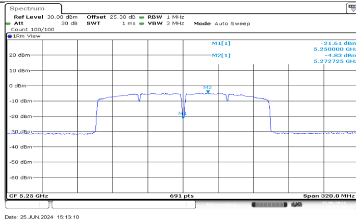
11AC160MIMO_Ant1_5250_UNII-2A
