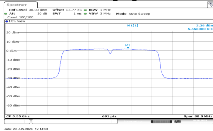
11AC40MIMO_Ant4_5550
