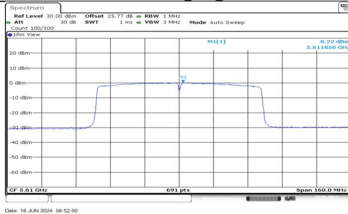
11AC80MIMO_Ant3_5610
