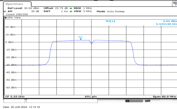
11AC40MIMO_Ant3_5550
