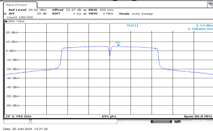
11AC40MIMO_Ant1_5795
