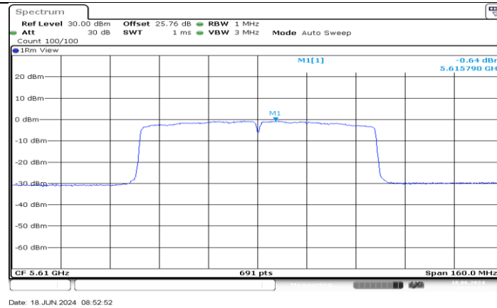
11AC80MIMO_Ant4_5610
