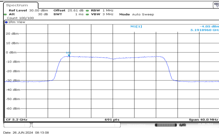
11AX20MIMO_Ant4_5200
