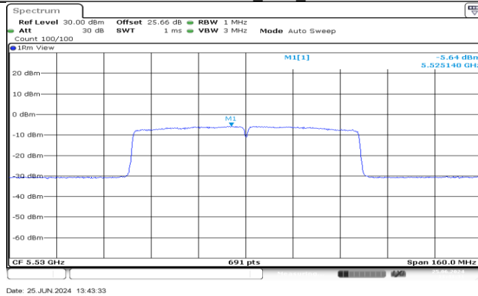
11AC80MIMO_Ant3_5530
