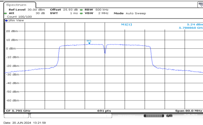
11AC40MIMO_Ant2_5795
