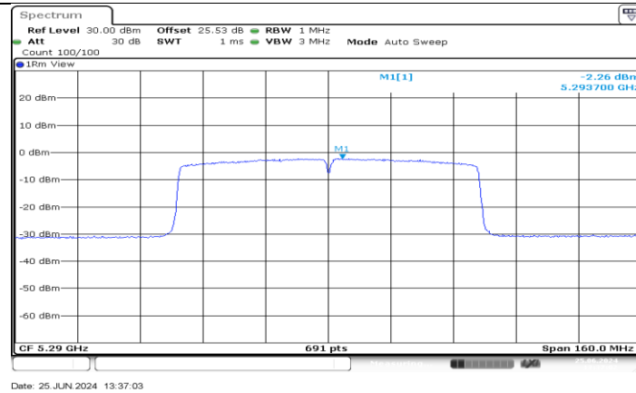
11AC80MIMO_Ant3_5290
