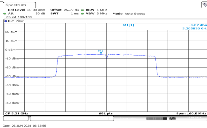
11AC80MIMO_Ant4_5210
