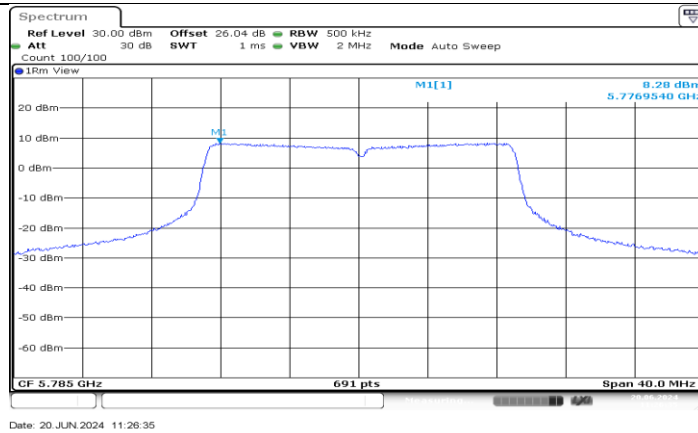
11AC20MIMO_Ant3_5785
