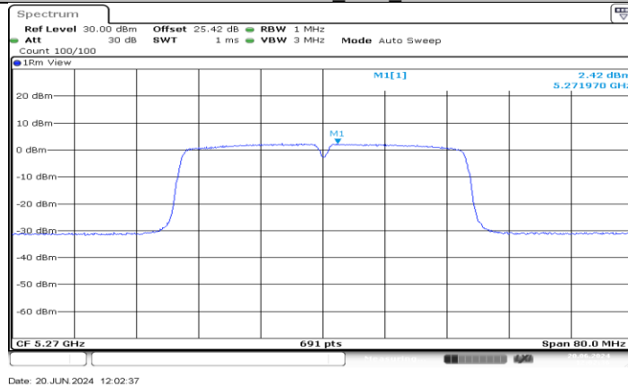
11AC40MIMO_Ant1_5270
