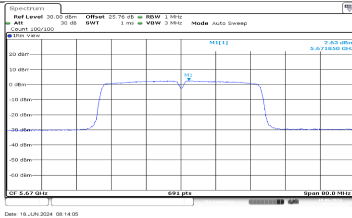
11AC40MIMO_Ant1_5670
