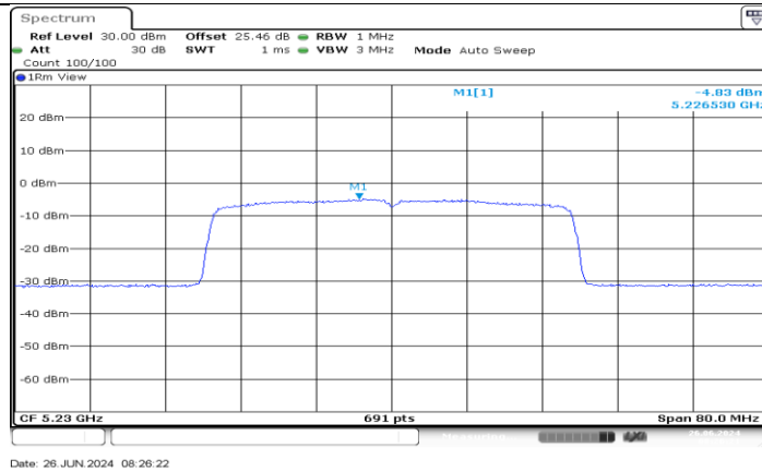
11AX40MIMO_Ant4_5230
