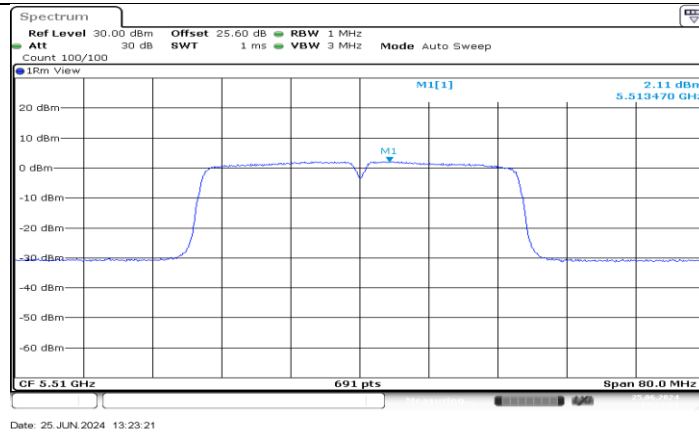
11AC40MIMO_Ant3_5510
