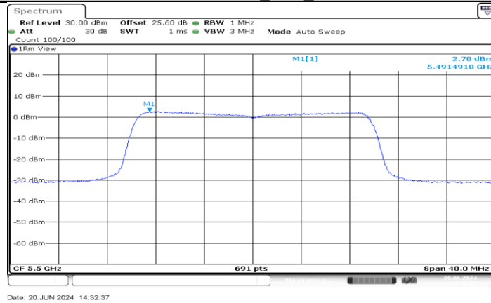
11AX20MIMO_Ant3_5500
