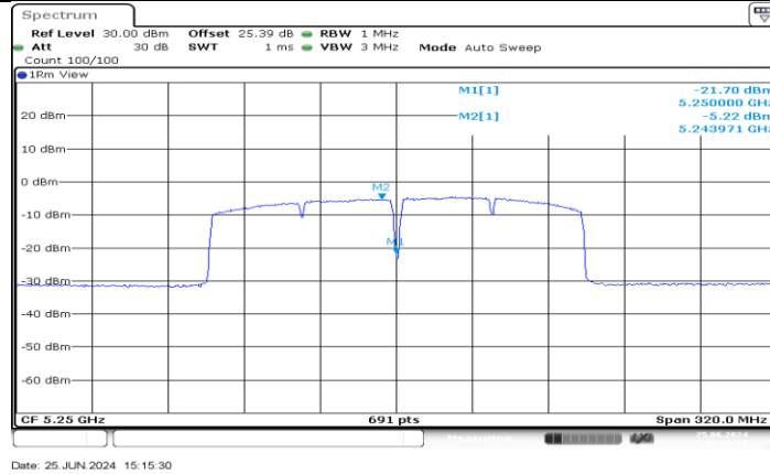
11AC160MIMO_Ant3_5250_UNII-1
