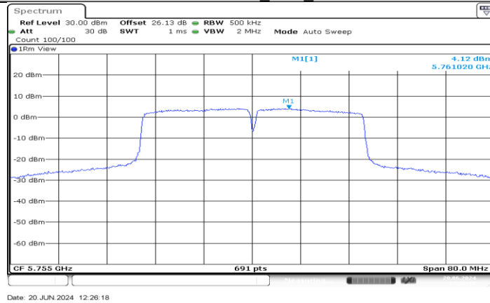
11AC40MIMO_Ant4_5755
