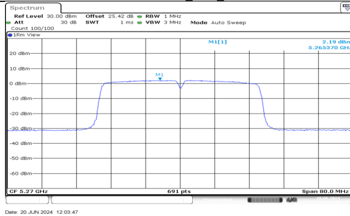
11AC40MIMO_Ant3_5270
