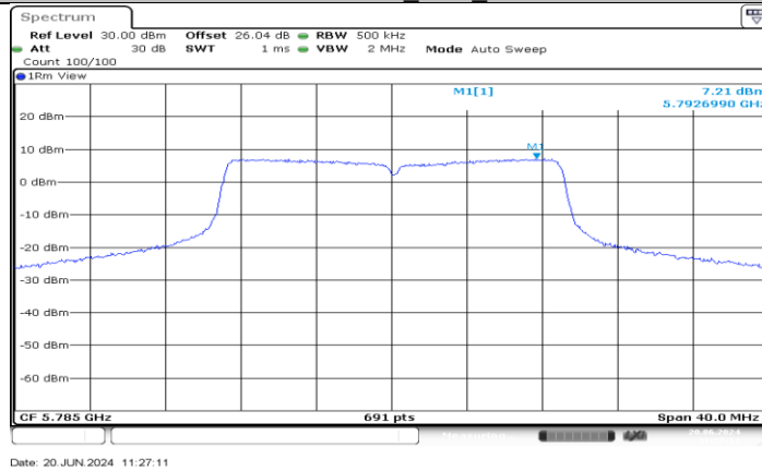
11AC20MIMO_Ant4_5785
