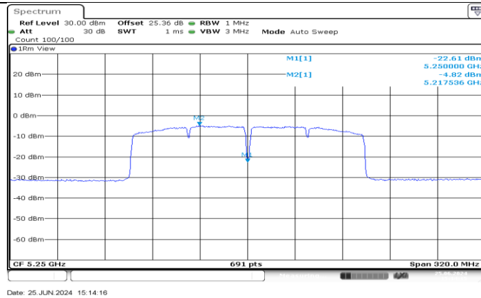
11AC160MIMO_Ant2_5250_UNII-1
