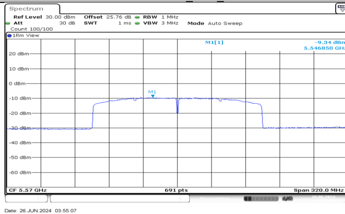
11AC160MIMO_Ant2_5570
