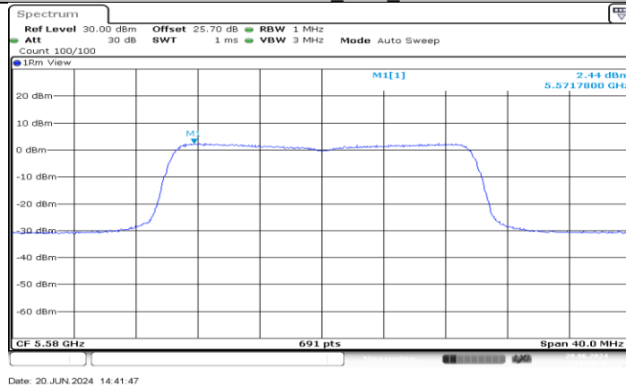
11AX20MIMO_Ant3_5580
