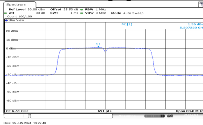
11AC40MIMO_Ant2_5510
