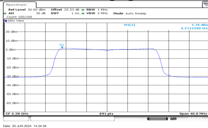
11AX20MIMO_Ant3_5280
