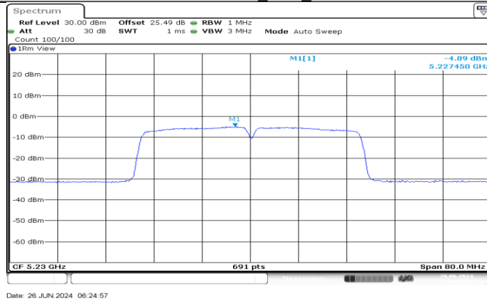
11AC40MIMO_Ant4_5230
