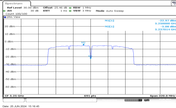
11AC160MIMO_Ant4_5250_UNII-1
