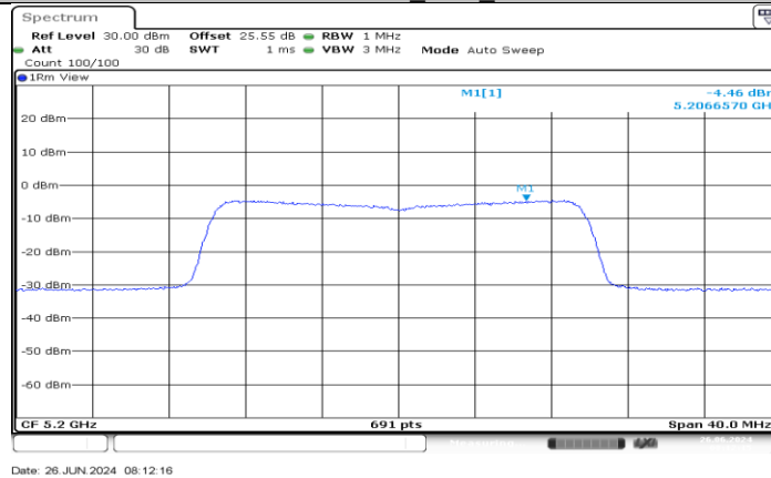
11AX20MIMO_Ant3_5200
