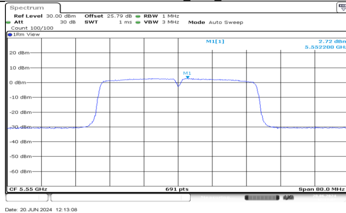
11AC40MIMO_Ant1_5550
