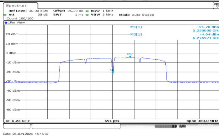
11AC160MIMO_Ant3_5250_UNII-2A
