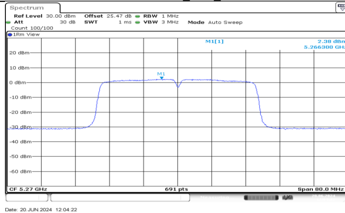
11AC40MIMO_Ant4_5270
