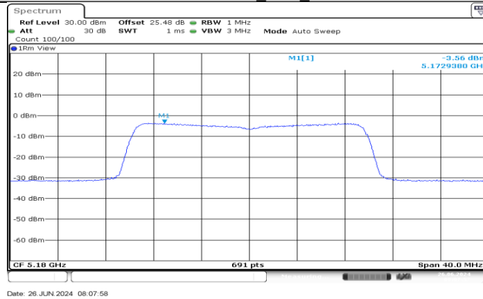
11AX20MIMO_Ant3_5180
