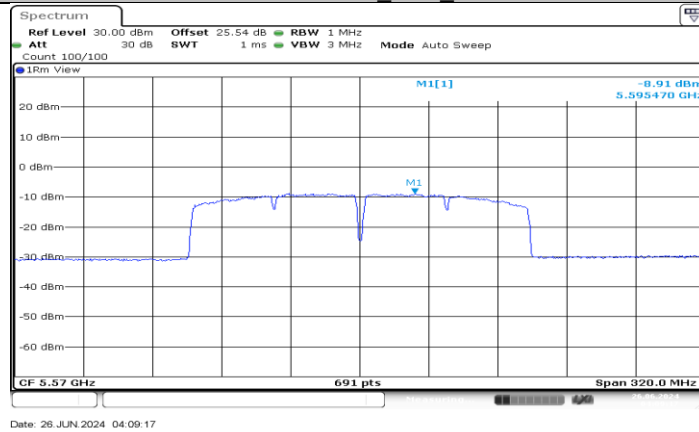
11AC160MIMO_Ant4_5570
