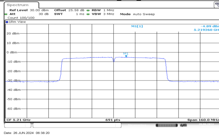
11AC80MIMO_Ant3_5210
