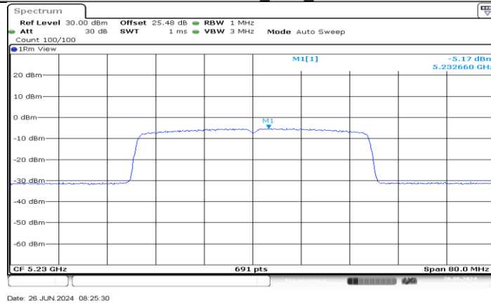
11AX40MIMO_Ant3_5230
