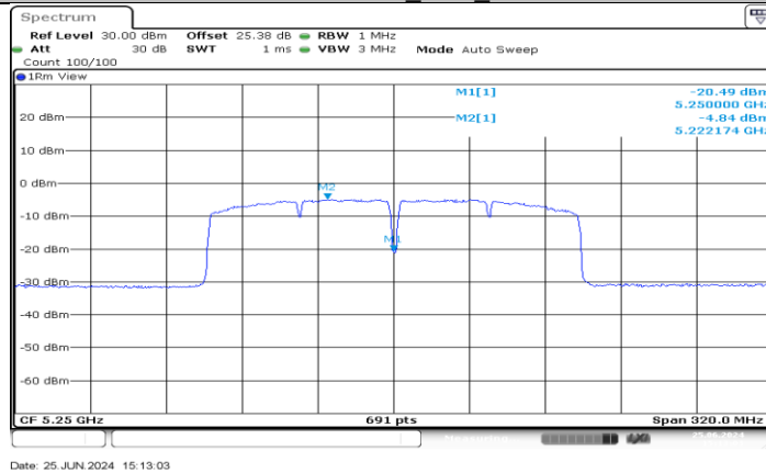
11AC160MIMO_Ant1_5250_UNII-1
