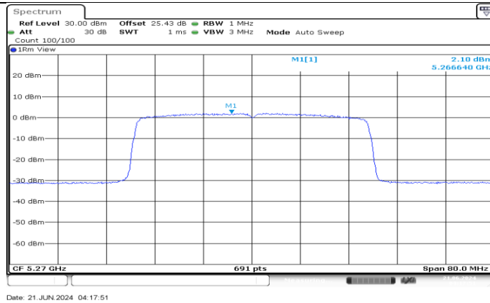
11AX40MIMO_Ant3_5270
