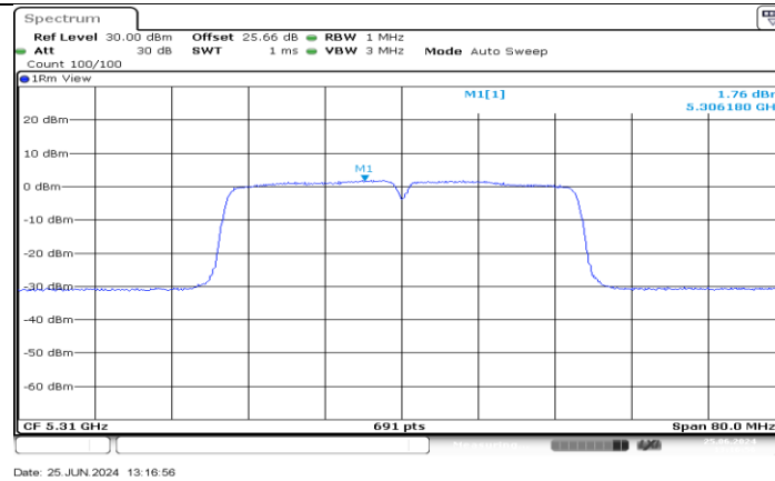
11AC40MIMO_Ant4_5310
