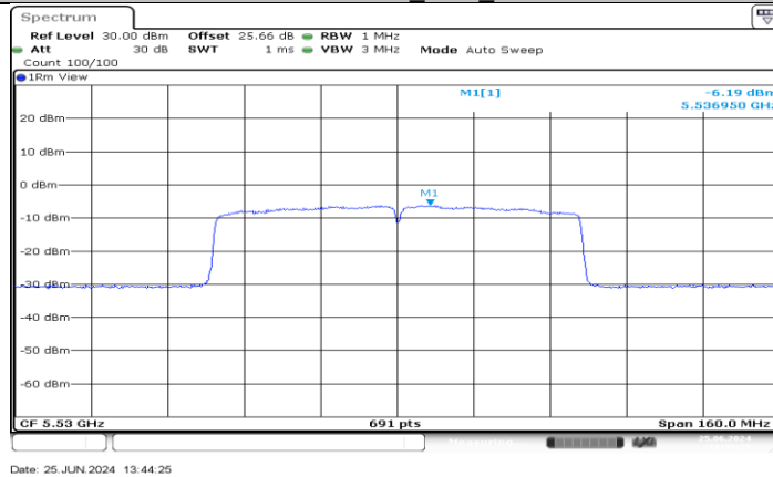
11AC80MIMO_Ant4_5530
