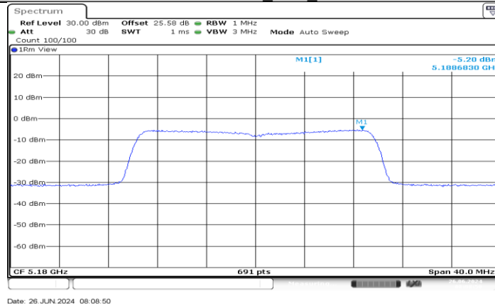
11AX20MIMO_Ant4_5180
