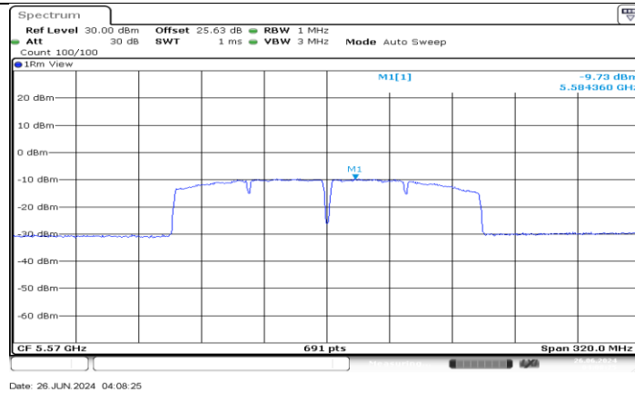
11AC160MIMO_Ant3_5570
