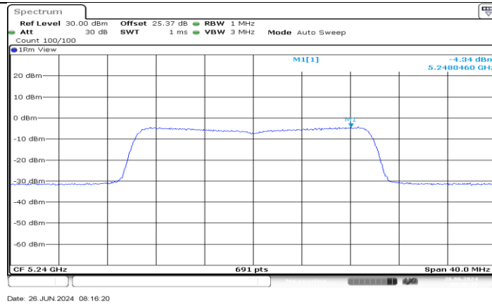
11AX20MIMO_Ant3_5240
