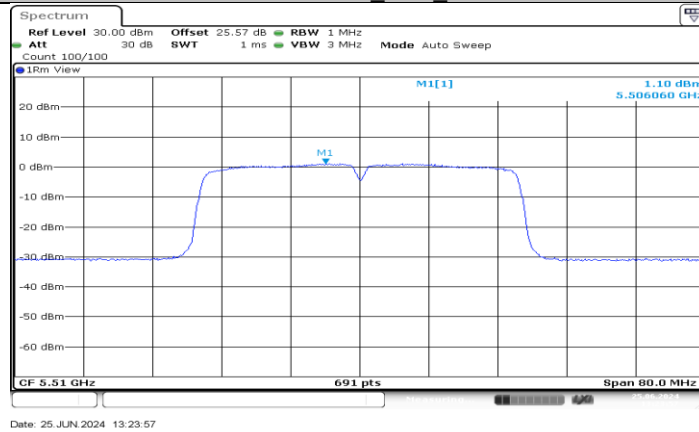
11AC40MIMO_Ant4_5510
