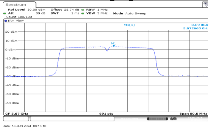
11AC40MIMO_Ant3_5670
