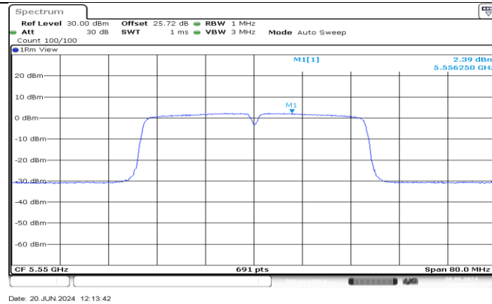
11AC40MIMO_Ant2_5550
