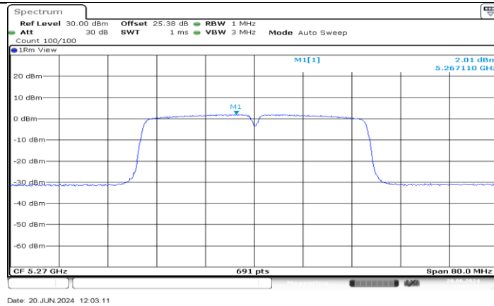
11AC40MIMO_Ant2_5270
