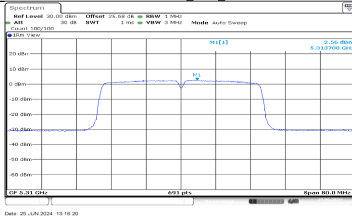
11AC40MIMO_Ant3_5310
