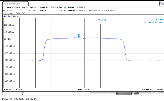
11AX40MIMO_Ant4_5270
