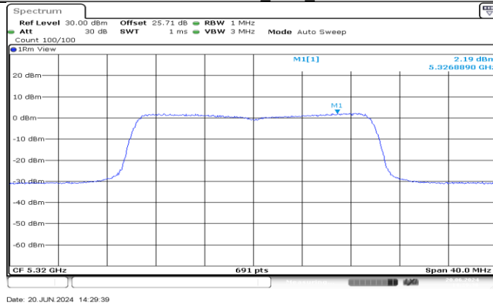
11AX20MIMO_Ant4_5320
