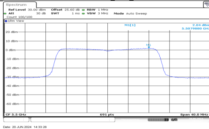
11AX20MIMO_Ant4_5500
