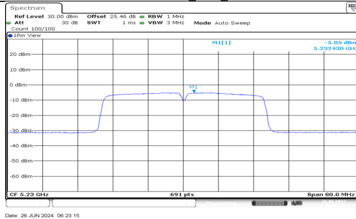
11AC40MIMO_Ant2_5230
