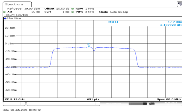
11AC40MIMO_Ant4_5190
