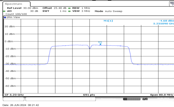
11AC40MIMO_Ant1_5230
