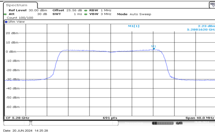
11AX20MIMO_Ant4_5280
