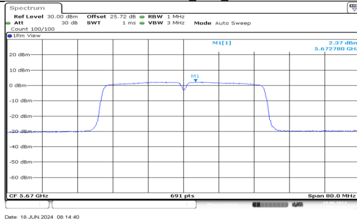
11AC40MIMO_Ant2_5670
