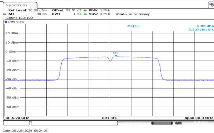
11AC40MIMO_Ant3_5230
