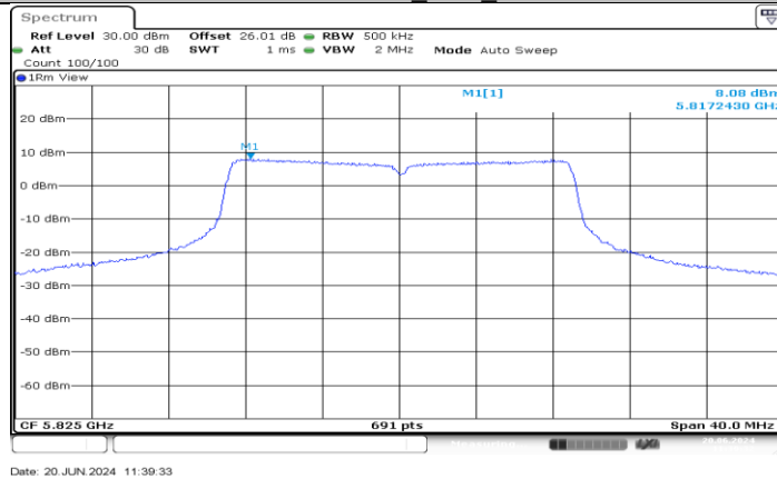
11AC20MIMO_Ant1_5825
