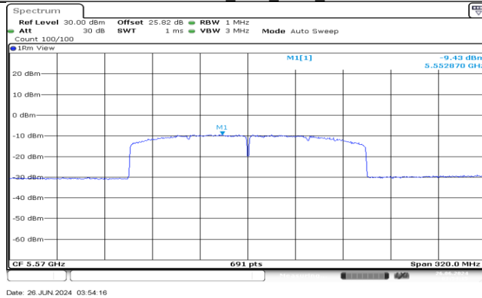
11AC160MIMO_Ant1_5570
