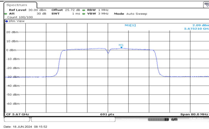
11AC40MIMO_Ant4_5670
