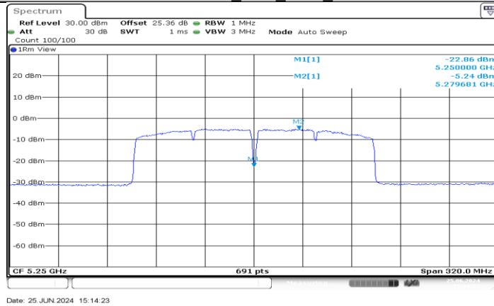
11AC160MIMO_Ant2_5250_UNII-2A
