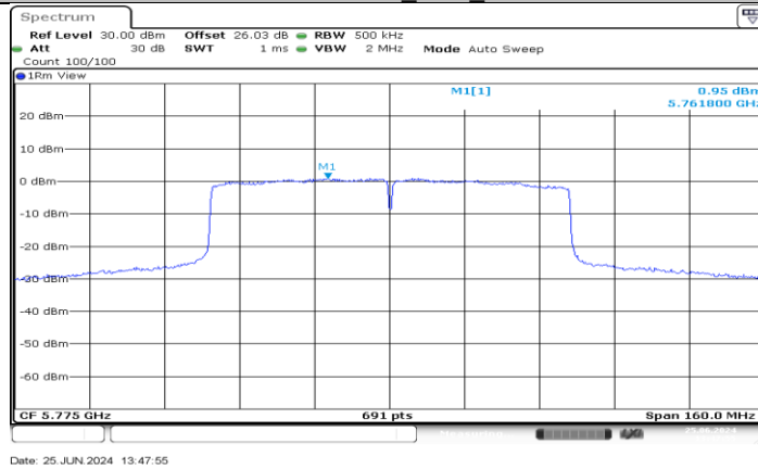
11AC80MIMO_Ant4_5775
