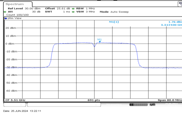
11AC40MIMO_Ant1_5510
