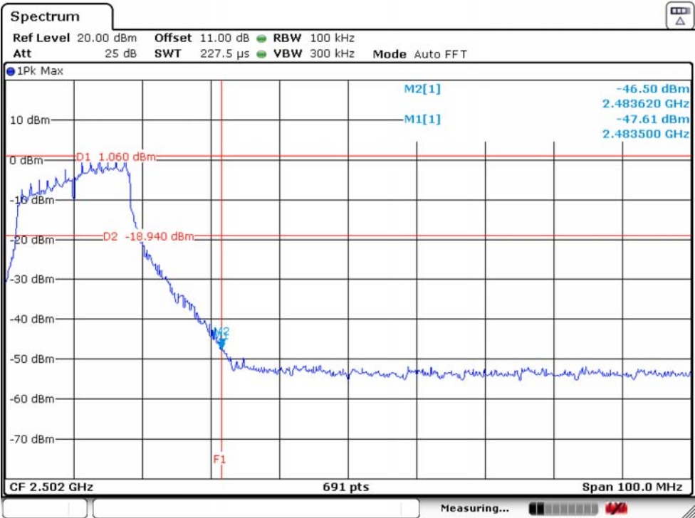
IEEE 802.11g 2462MHz
