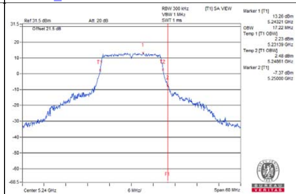
802.11a_Chain 1 / CH48
