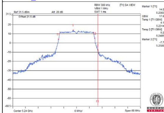
802.11a_Chain 2 / CH48
