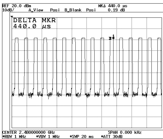
CH 78 2480MHz
