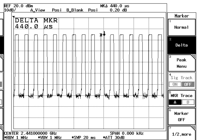
CH 39 2441MHz
