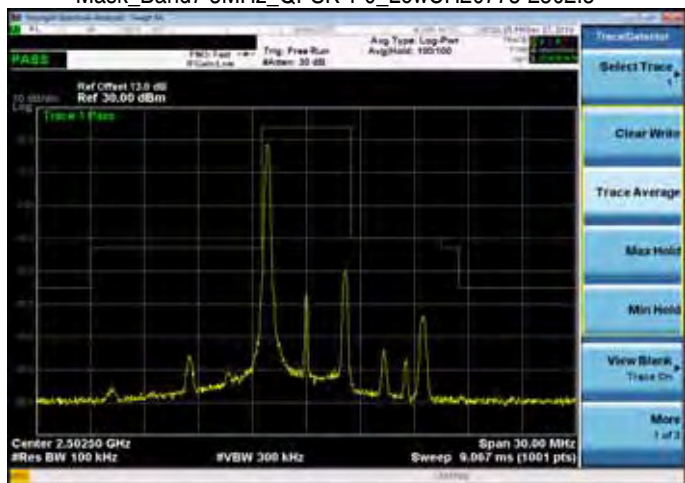
Mask_Band7 5MHz_QPSK 1 0_LowCH20775-2502.5
