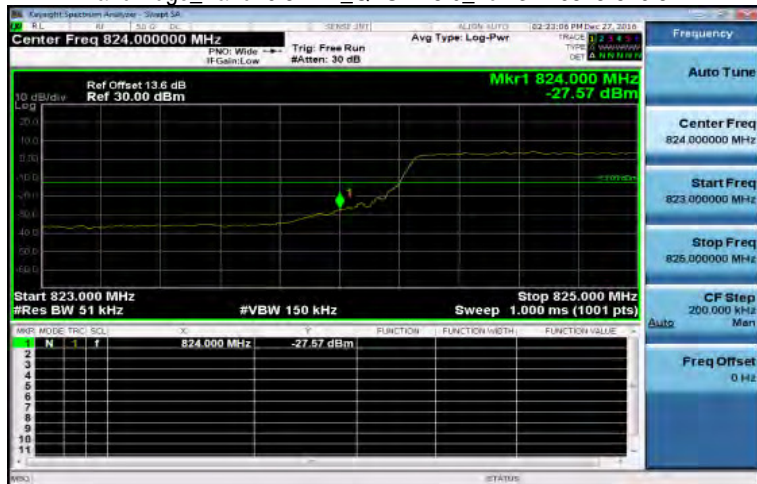
Band Edge_Band26 5MHz_QPSK 25 0_LowCH26815-826.5
