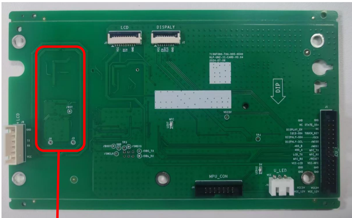
RFID Antenna
