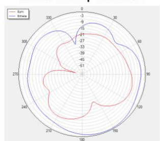
Theta=90 freq=2500MHz
