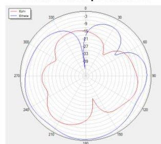
Theta=90 freq=2400MHz
