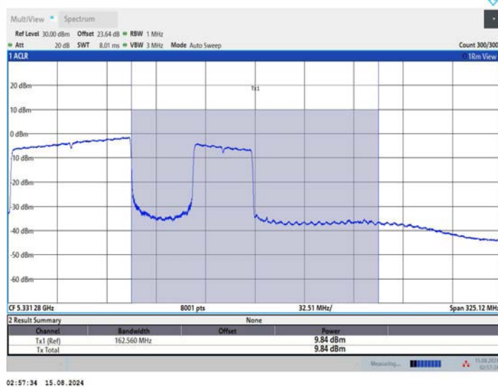
11BE160MIMO_Ant2_5250_UNII-2A_996+484_OFDMA_4
