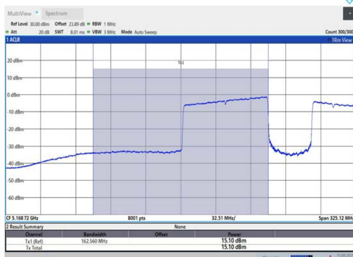
11BE160MIMO_Ant2_5250_UNII-1_996+484_OFDMA_4
