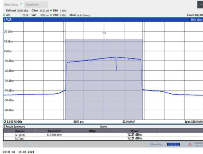
11BE160MIMO Ant1 5570 996+484 OFDMA 4
