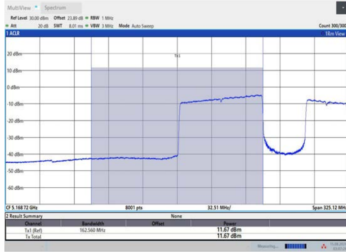
11BE160MIMO_Ant2_5250_UNII-1_996+484_OFDMA_3
