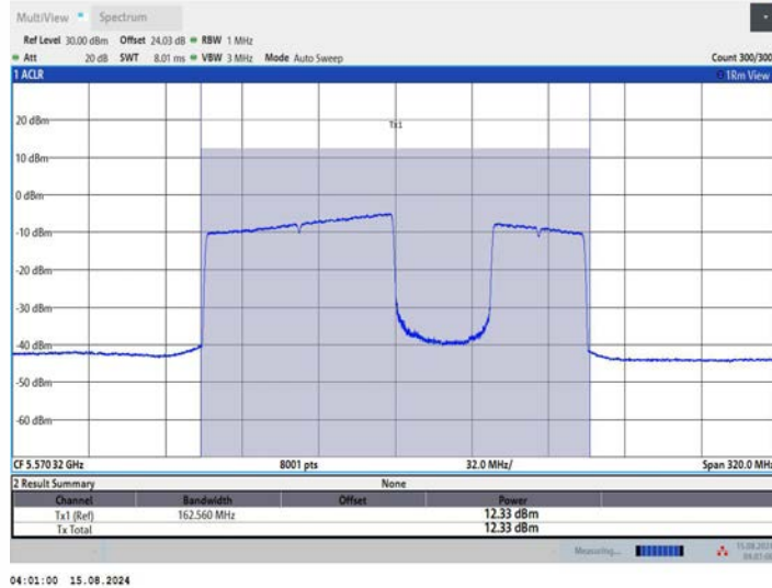
11BE160MIMO Ant1 5570 996+484 OFDMA 3
