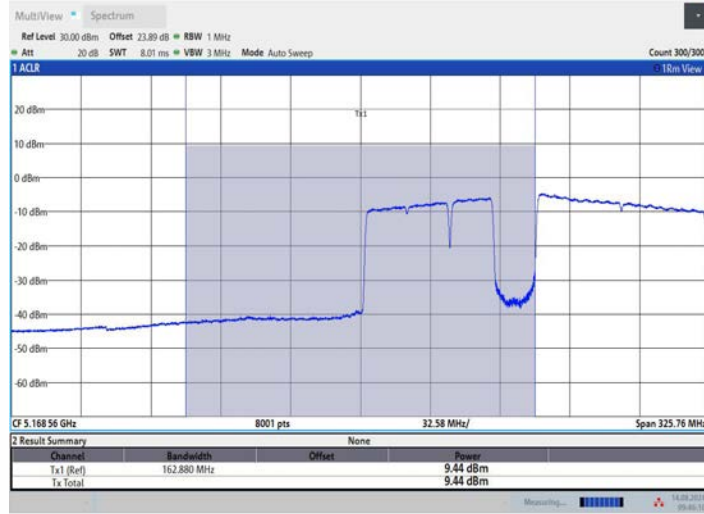
11BE160MIMO_Ant2_5250_UNII-1_996+484+242_OFDMA_4
