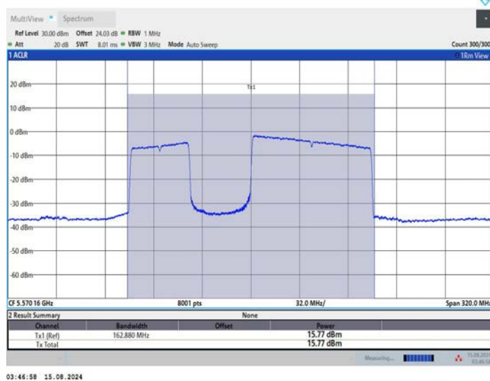
11BE160MIMO Ant1 5570 996+484 OFDMA 3
