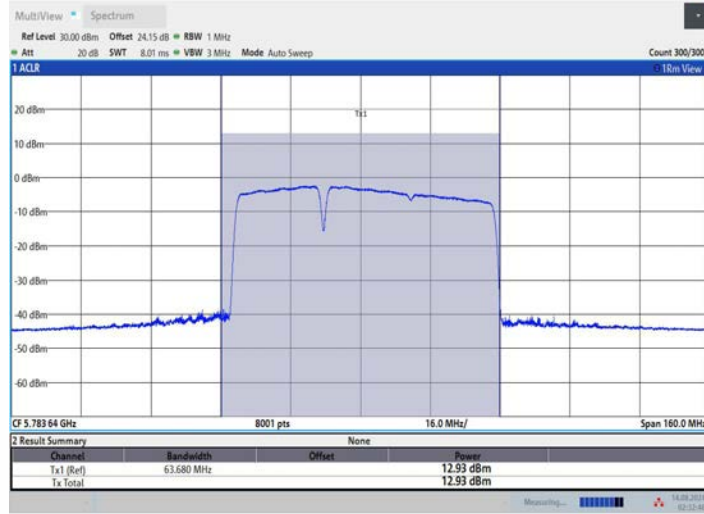
11BE80MIMO_Ant2_5775_484+242_OFDMA_2
