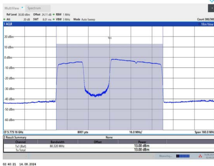
11BE80MIMO_Ant2_5775_484+242_OFDMA_3
