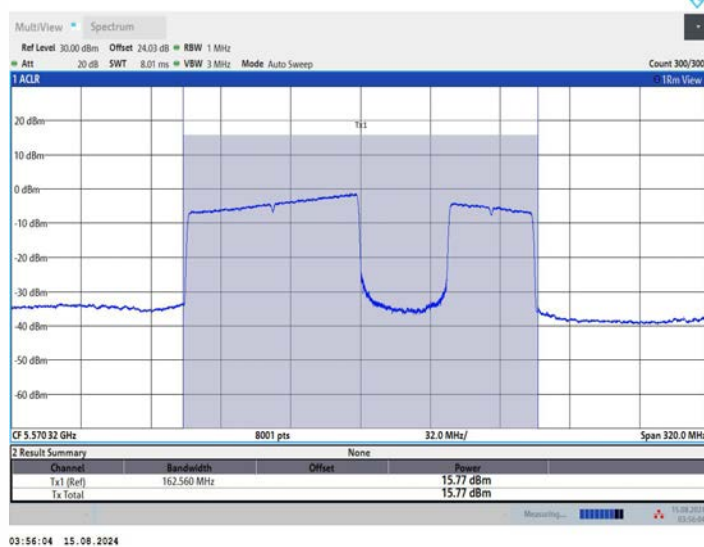
11BE160MIMO Ant1 5570 996+484 OFDMA 4
