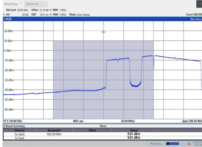
11BE160MIMO_Ant3_5250_UNII-1_996+484+242_OFDMA_3
