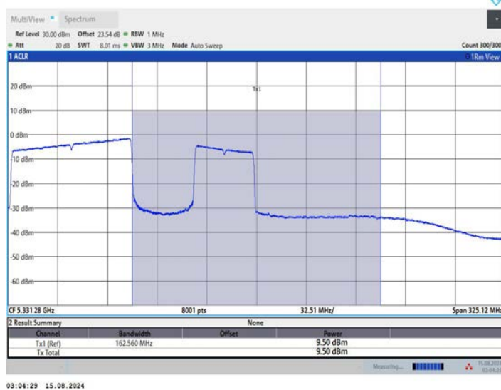
11BE160MIMO_Ant3_5250_UNII-2A_996+484_OFDMA_4
