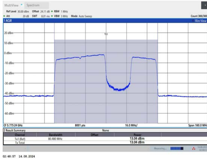
11BE80MIMO_Ant2_5775_484+242_OFDMA_4
