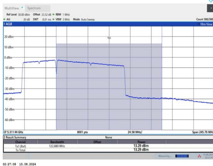
11BE160MIMO Ant1 5250 UNII-2A 996+484 OFDMA_2
