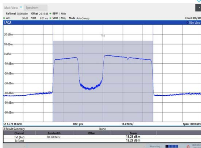
11BE80MIMO_Ant3_5775_484+242_OFDMA_3
