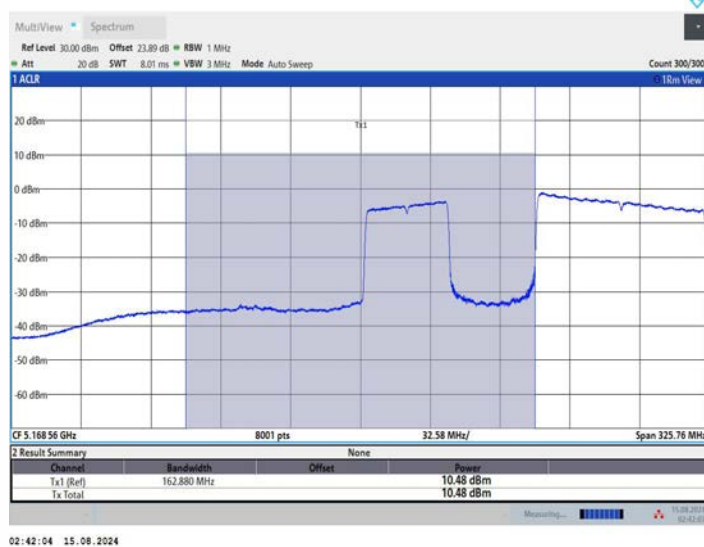
11BE160MIMO_Ant2_5250_UNII-1_996+484_OFDMA_3
