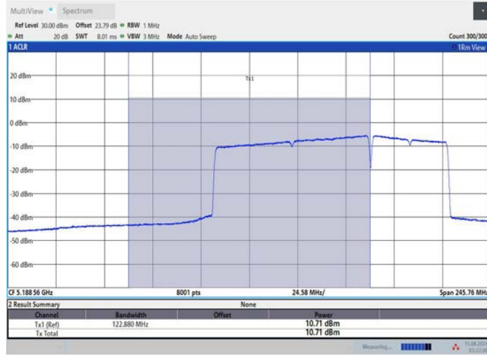
11BE160MIMO_Ant3_5250_UNII-1_996+484_OFDMA_4
