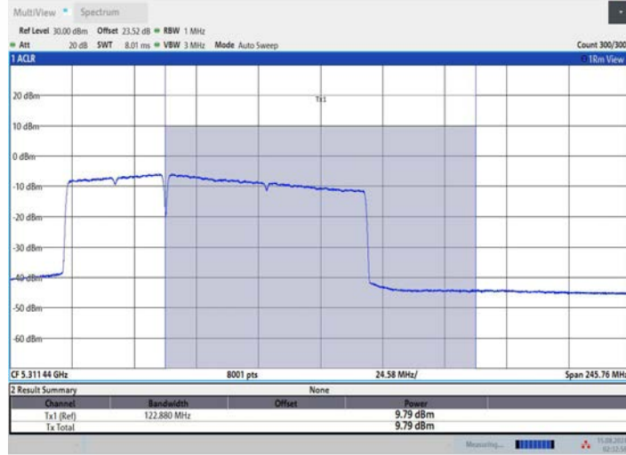
11BE160MIMO Ant1 5250 UNII-2A 996+484 OFDMA_1
