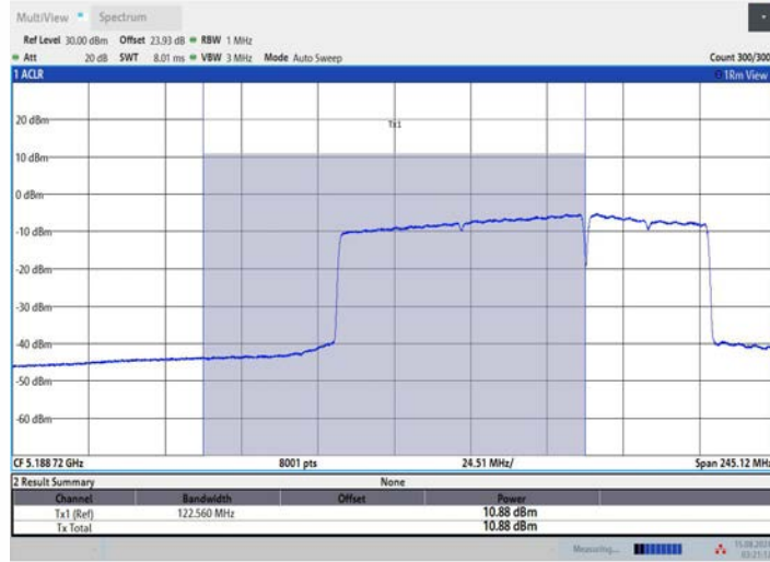
11BE160MIMO_Ant2_5250_UNII-1_996+484_OFDMA_4
