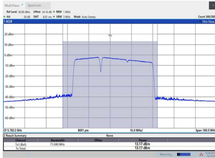
11BE80MIMO_Ant3_5775_484+242_OFDMA_2
