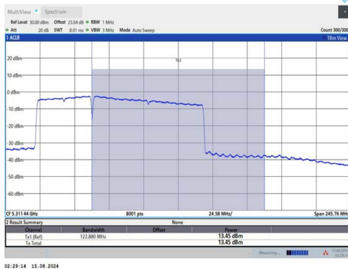
11BE160MIMO Ant2 5250 UNII-2A 996+484 OFDMA_2
