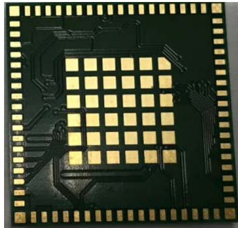
Bottom
