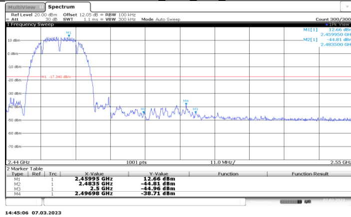
11B-CDD_Ant1_High_2457
