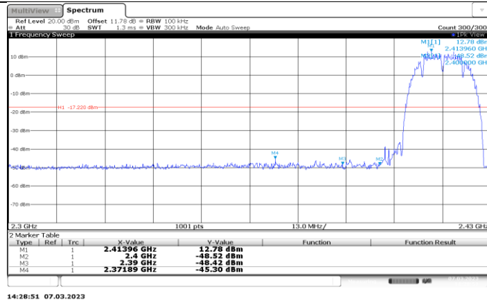
11B-CDD_Ant5_Low_2417
