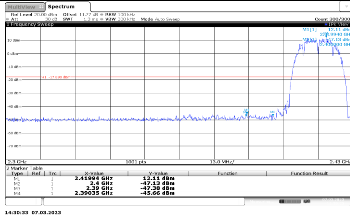
11B-CDD_Ant7_Low_2417
