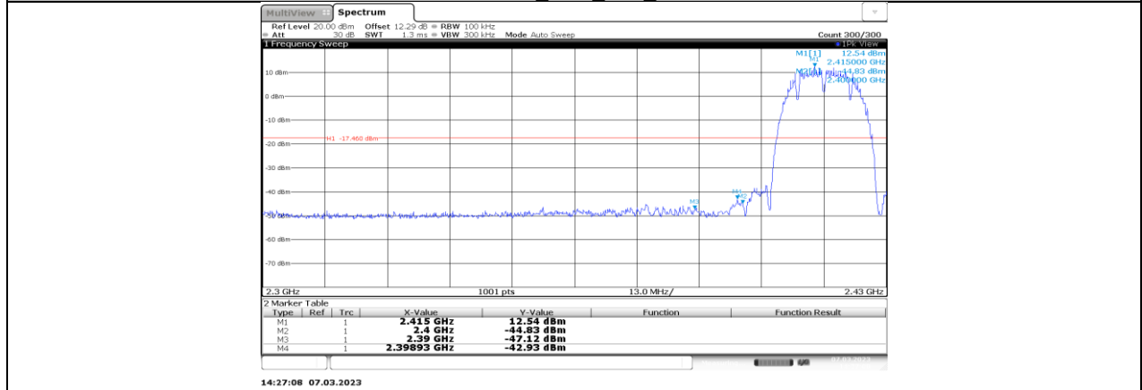
11B-CDD_Ant3_Low_2417
