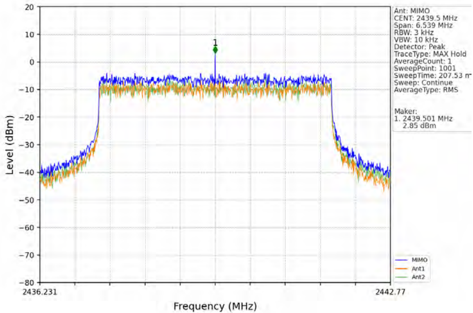
5M_MCH_2439.5MHz_MIMO_NTNV
