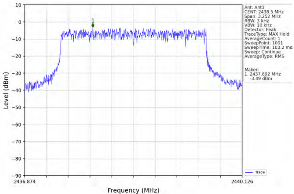
3M_MCH_2438.5MHz_Ant3_NTNV
