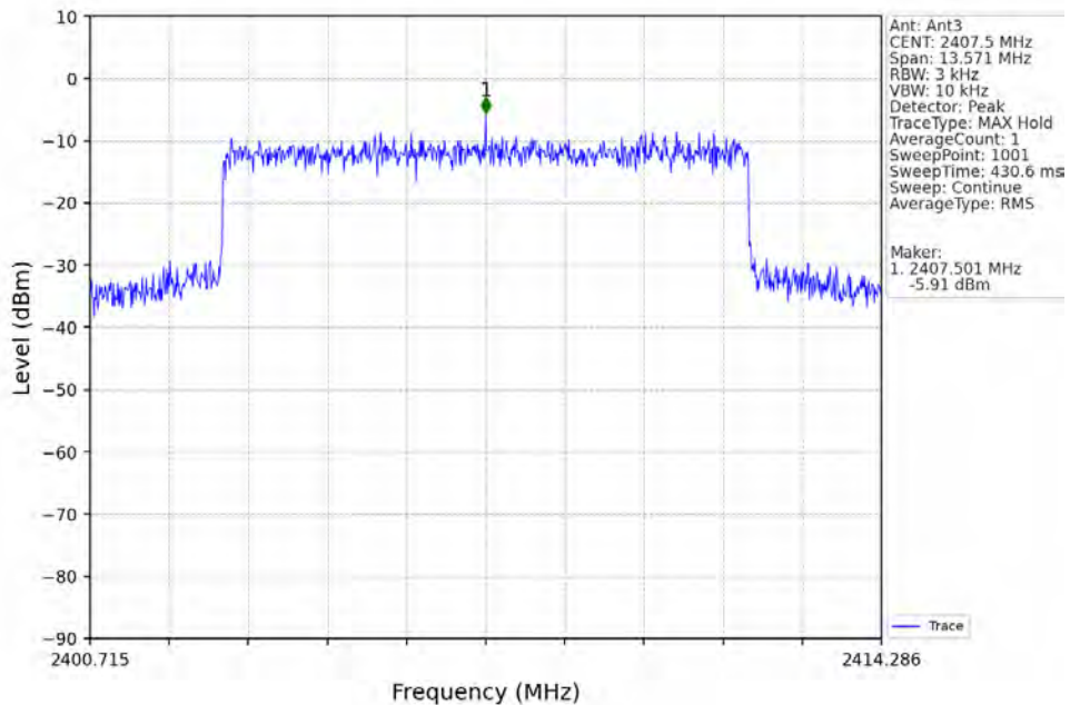
10M_LCH_2407.5MHz_MIMO_NTNV
