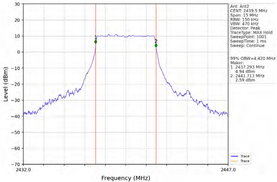
5M_MCH_2439.5MHz_Ant2_NTNV
