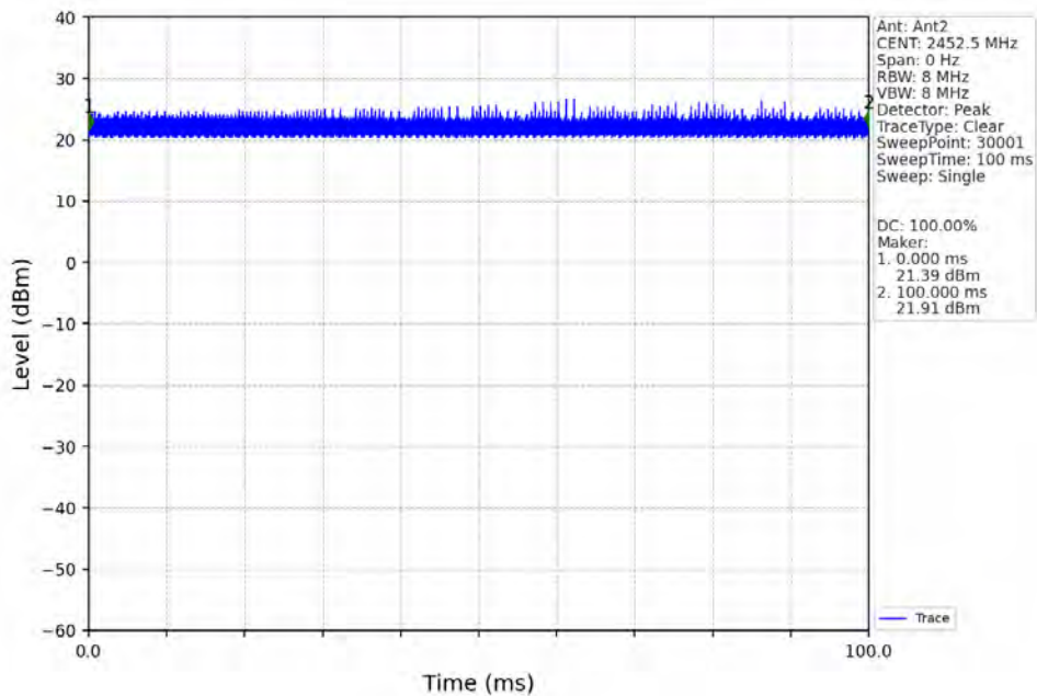
40M_HCH_2452.5MHz_Ant2_NTNV
