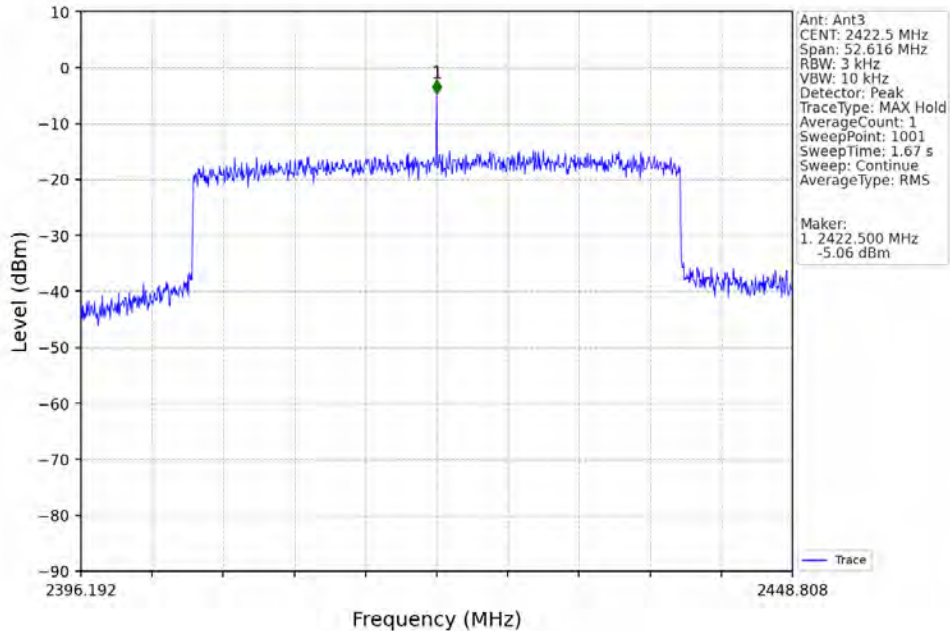
40M_LCH_2422.5MHz_MIMO_NTNV
