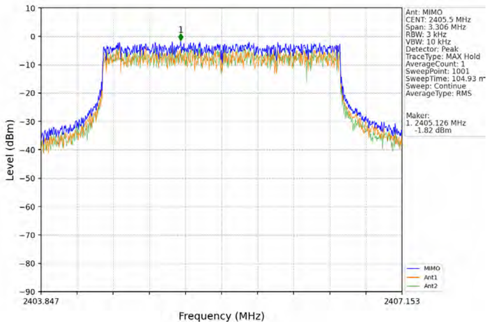
3M_LCH_2405.5MHz_MIMO_NTNV
