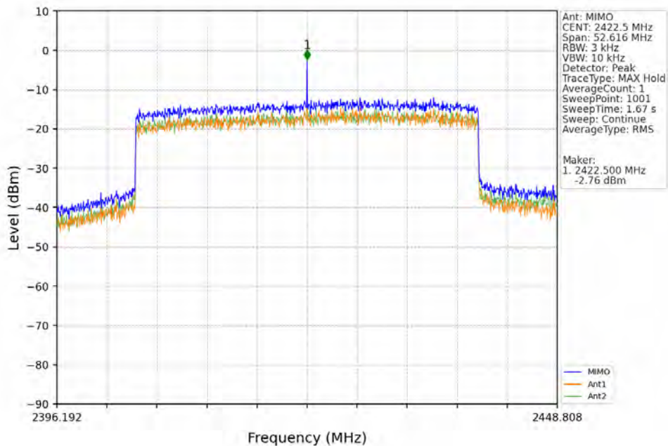
40M_LCH_2422.5MHz_MIMO_NTNV
