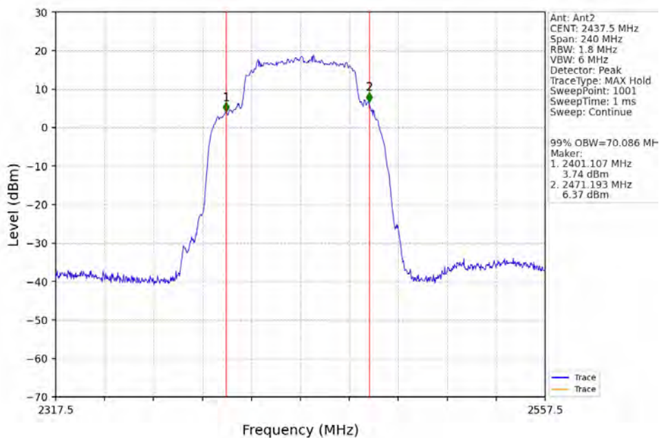
60M_MCH_2437.5MHz_Ant2_NTNV
