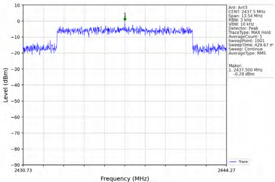
10M_MCH_2437.5MHz_Ant3_NTNV
