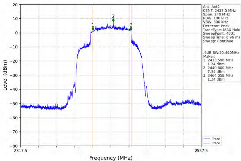
60M_MCH_2437.5MHz_Ant2_NTNV
