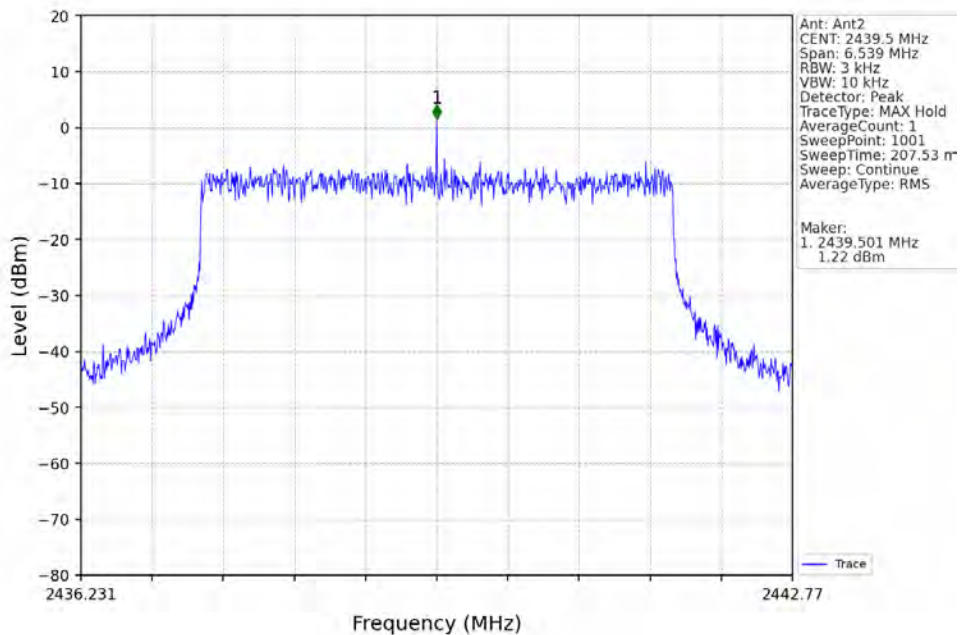
5M_MCH_2439.5MHz_Ant2_NTNV
