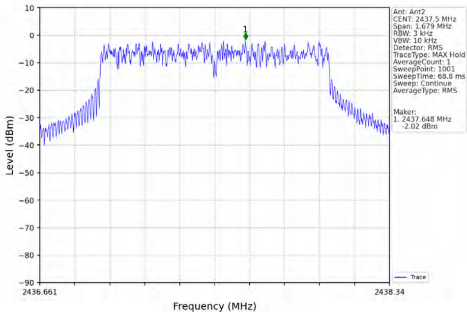
1.4M_MCH_2437.5MHz_Ant2_NTNV
