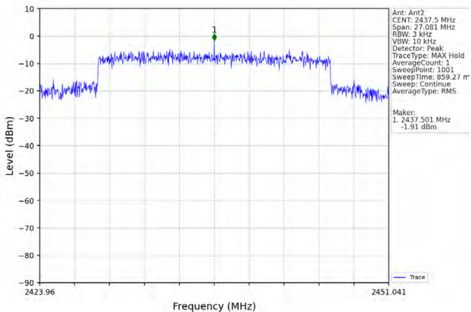
20M_MCH_2437.5MHz_Ant2_NTNV
