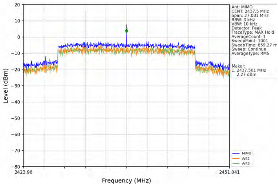
20M_MCH_2437.5MHz_MIMO_NTNV
