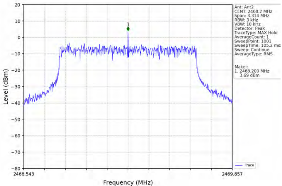
3M_HCH_2468.2MHz_Ant2_NTNV
