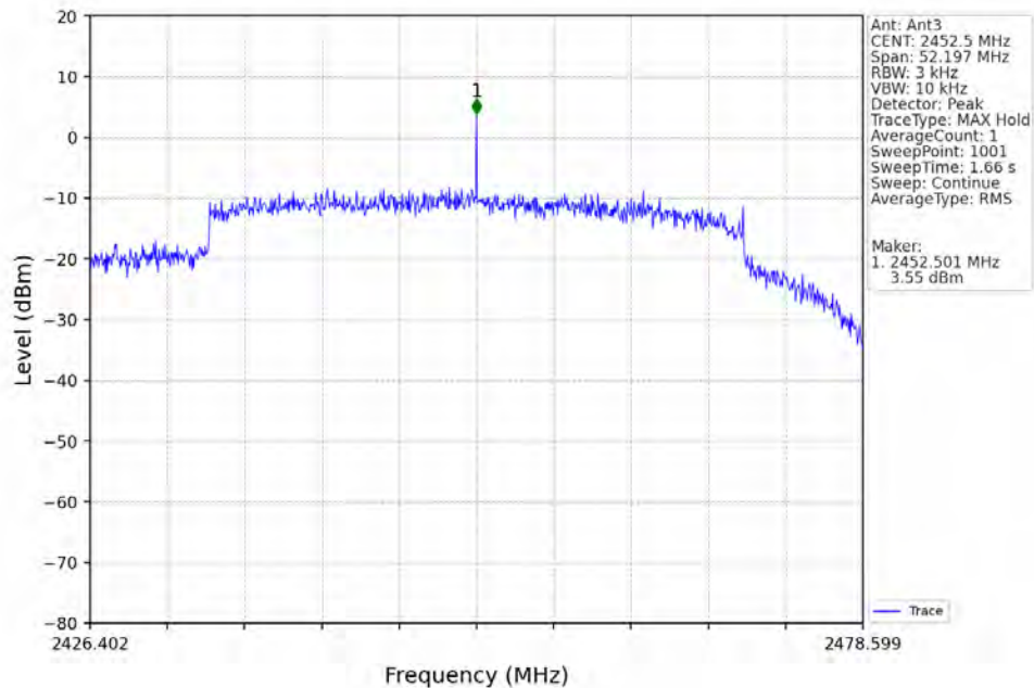
40M_HCH_2452.5MHz_MIMO_NTNV
