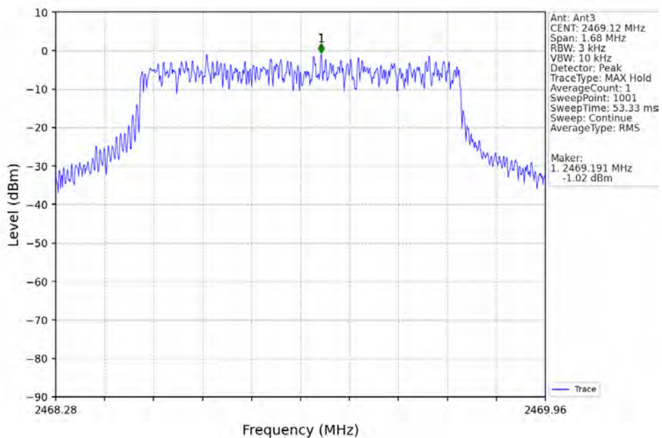
1.4M_HCH_2469.12MHz_Ant3_NTNV
