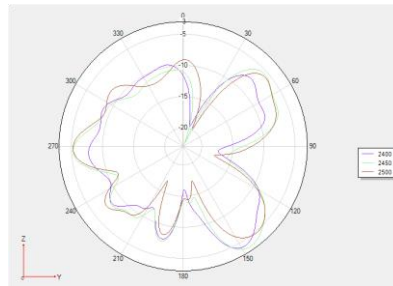
Phi 90 2D 图
