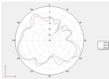
Phi 0 2D 图
